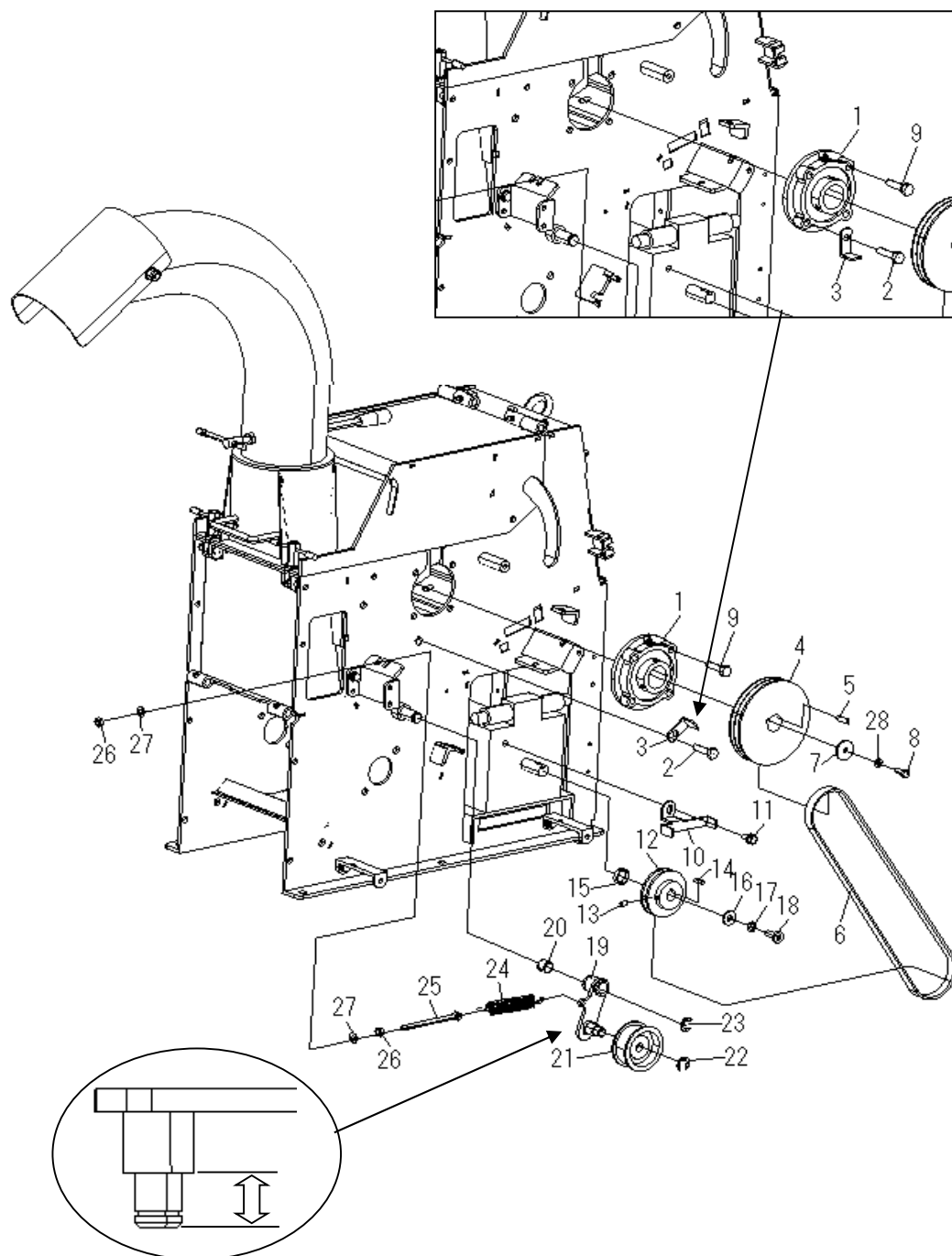
19番 Bテンションアーム
