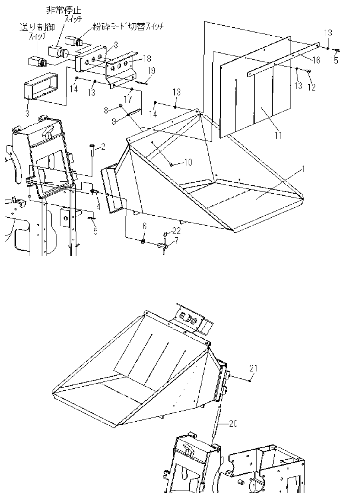
Fig. 12 ホツパ系
