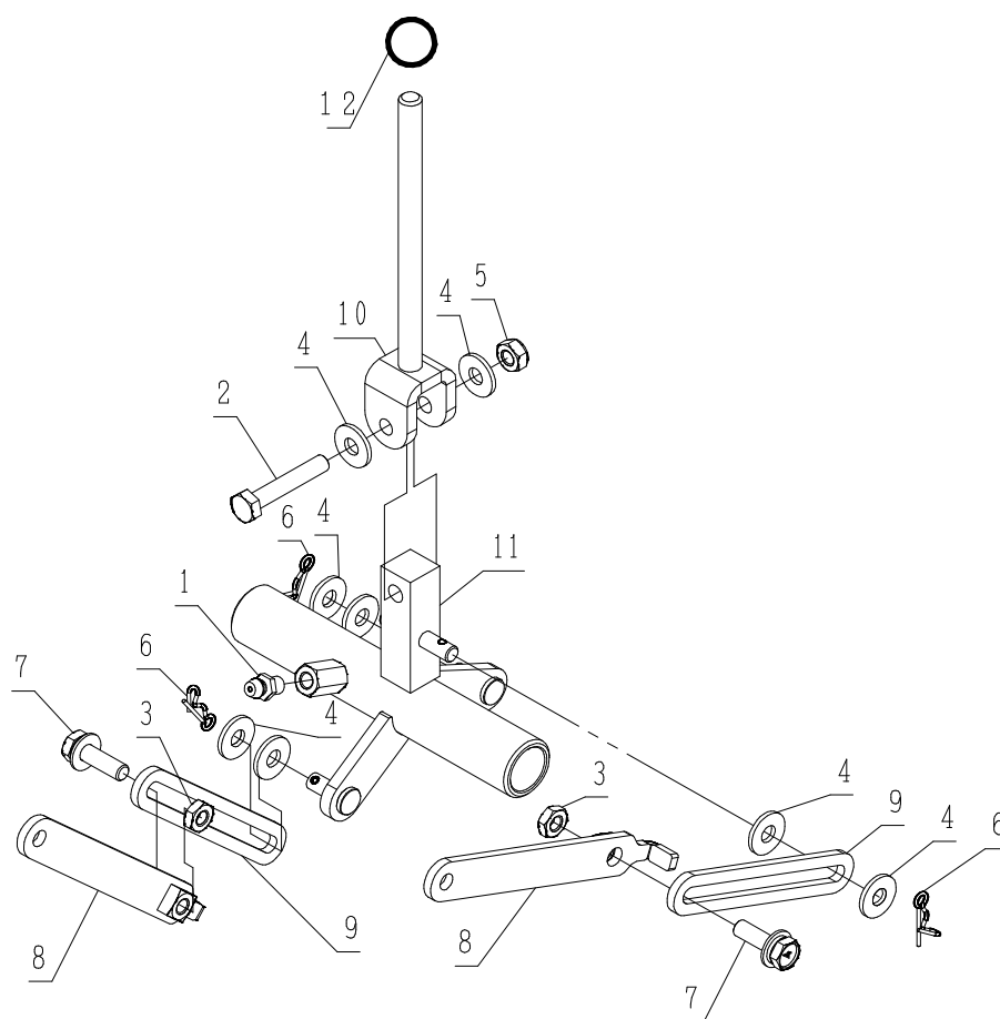
Fig. 9 走行レバーアームSub組
