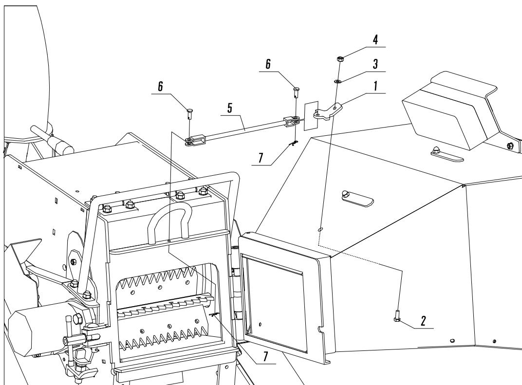
Fig. 28 ホツパ3
