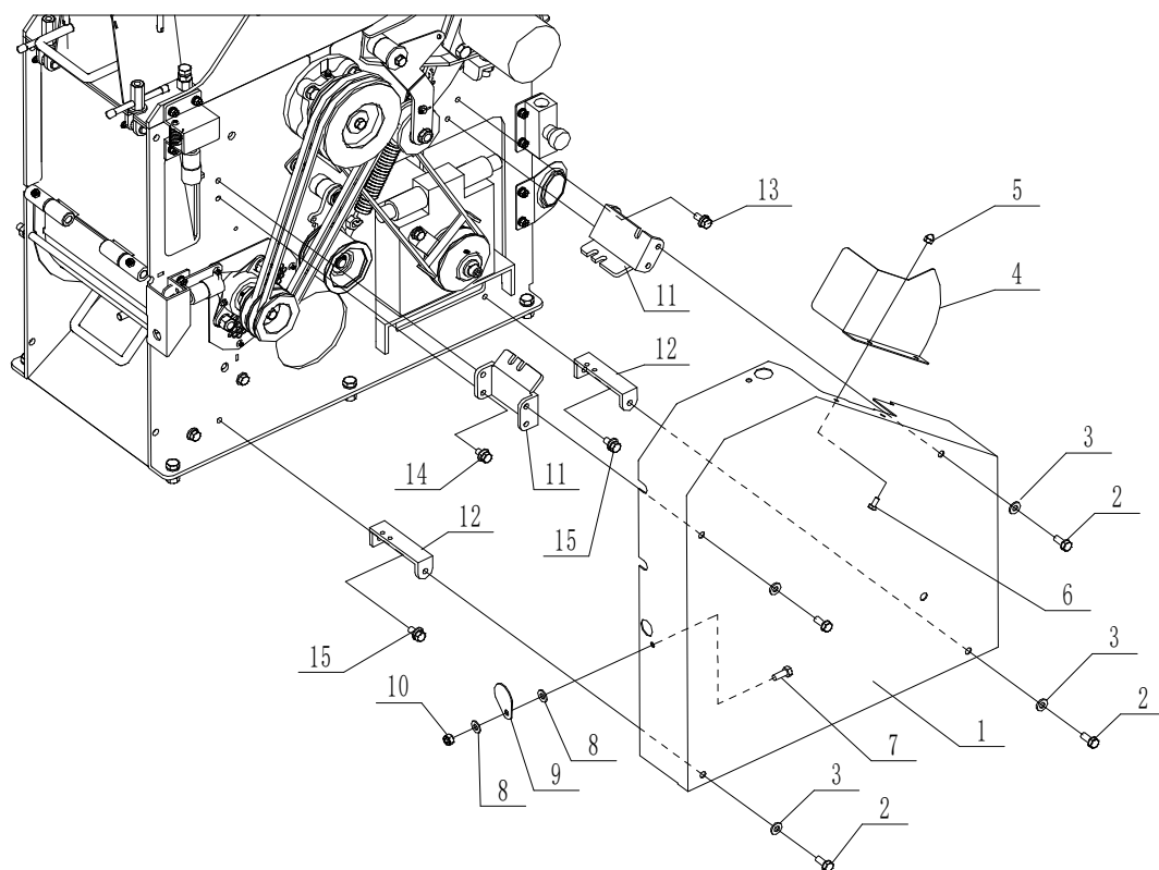
Fig. 31 カバーL
