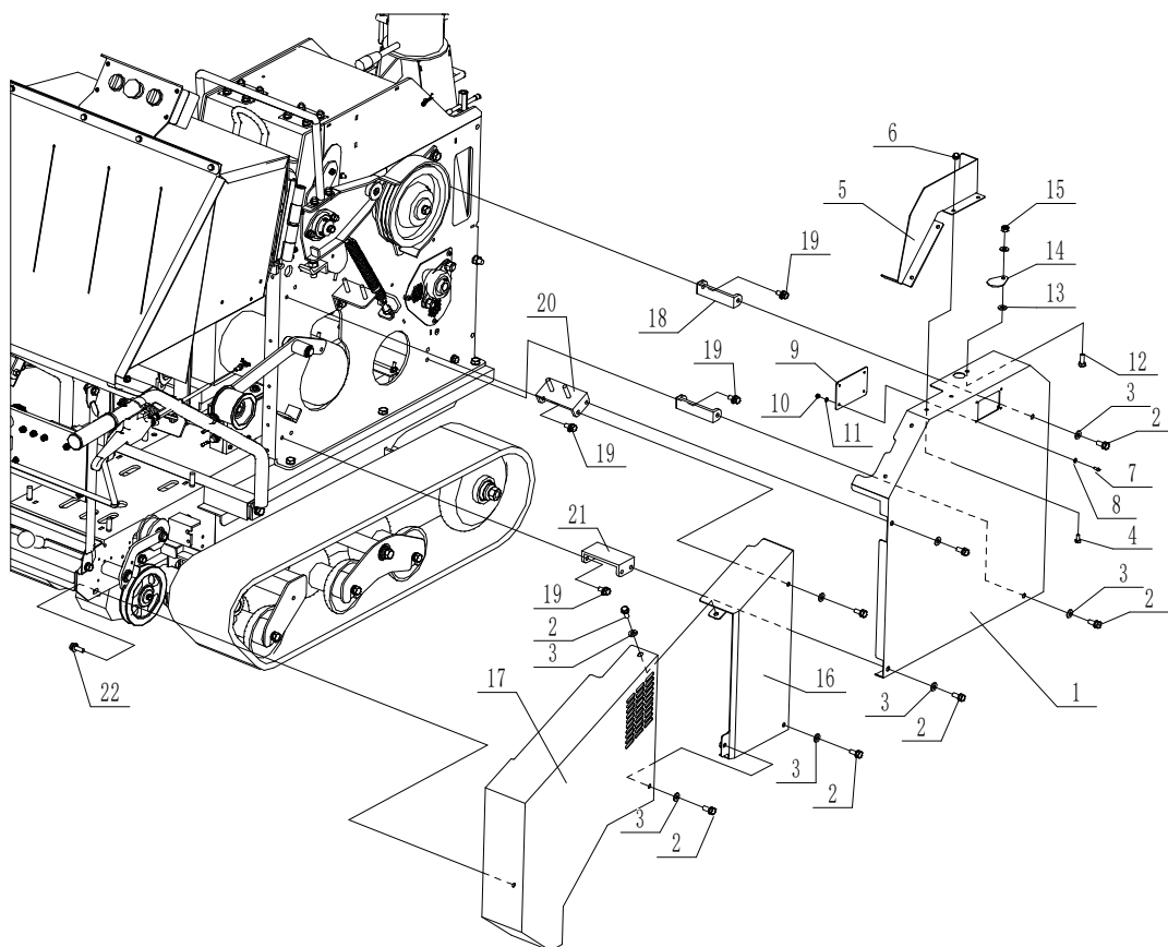
Fig. 30 カバー-R
