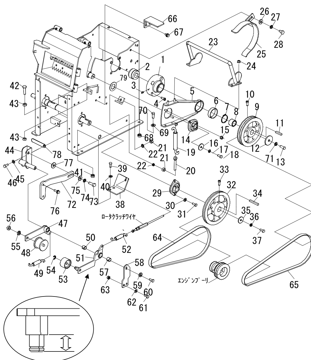
Fig. 8 ロータハウジングR系
