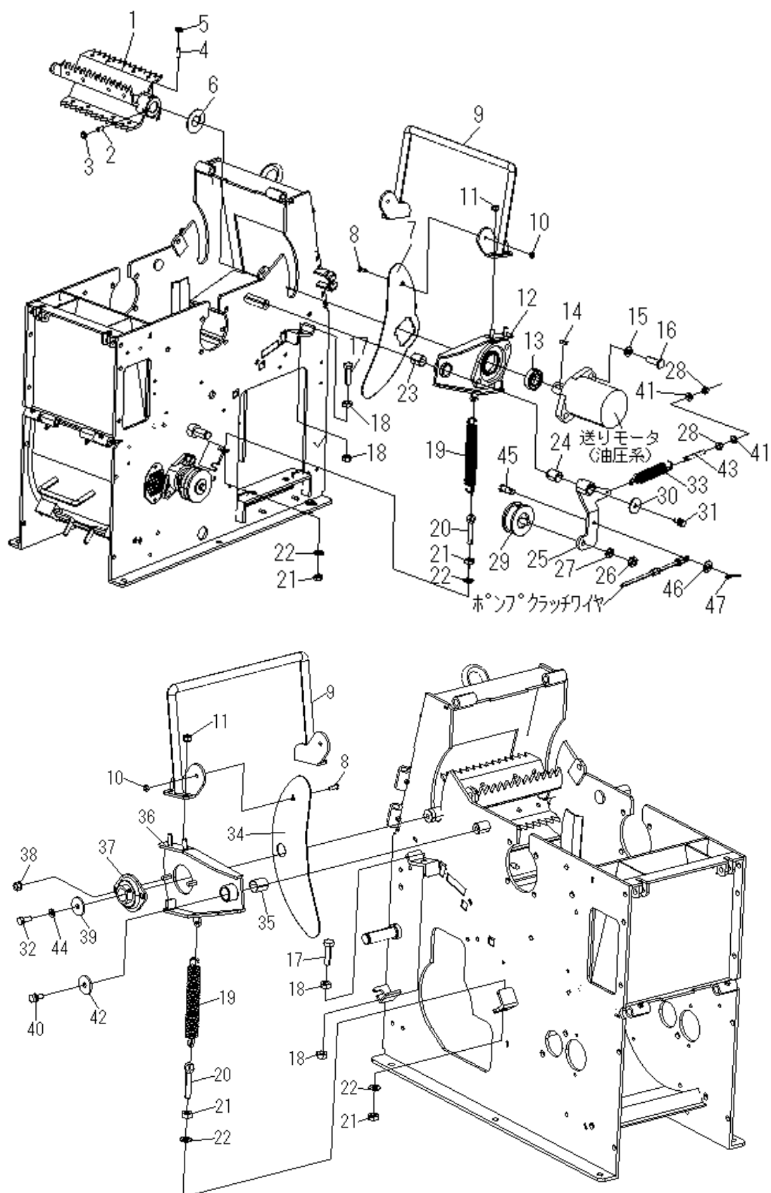
Fig. 11 フィーダ系
