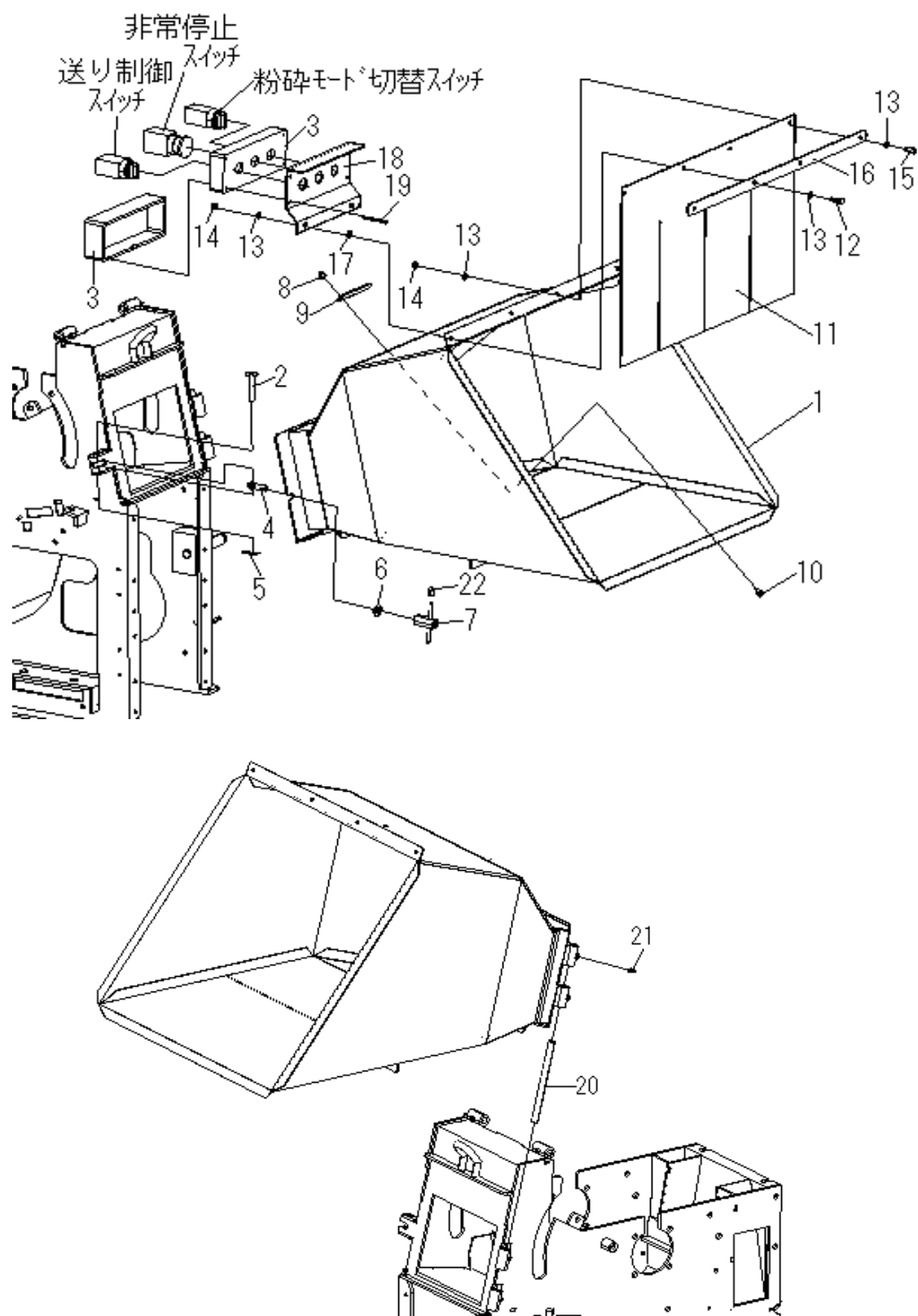
Fig. 12 ホツパ系
