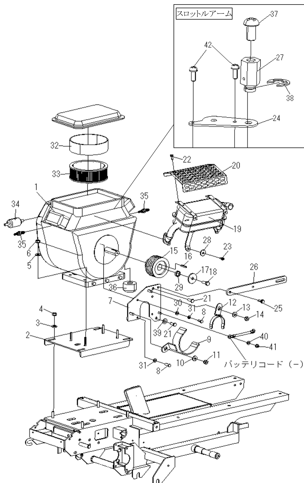
Fig. 4 エンジン系
