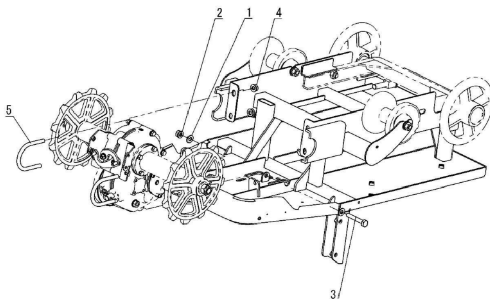
Fig. 8 シャーシ③
