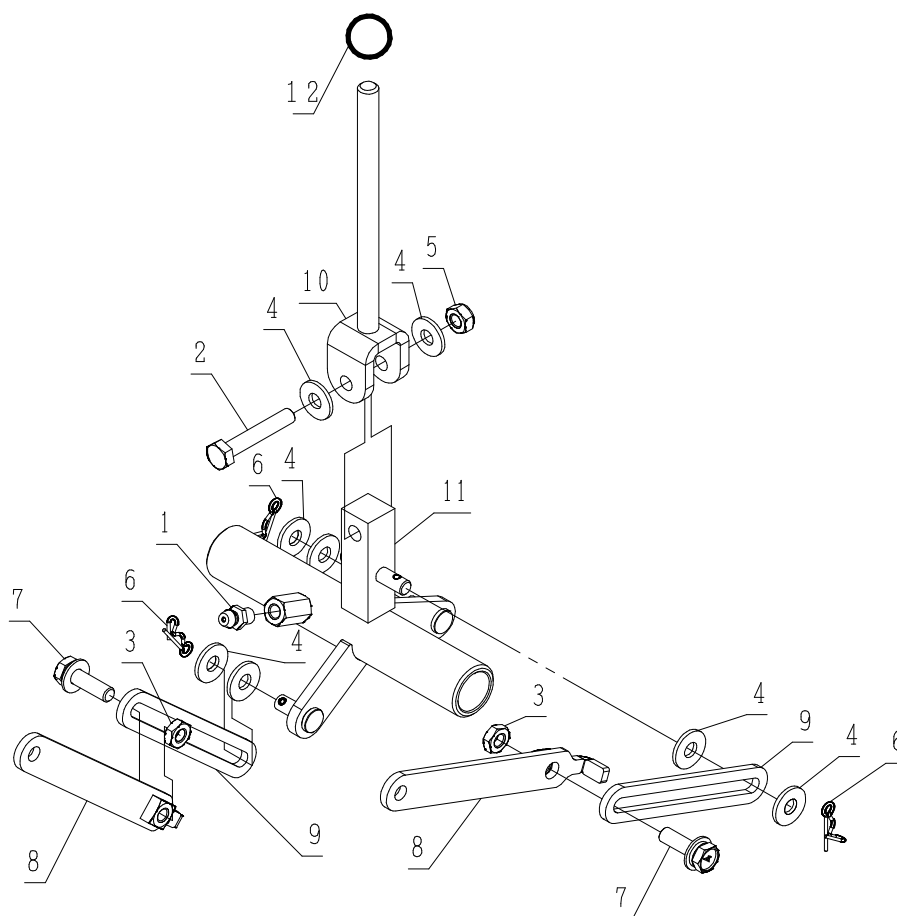
Fig. 9 走行レバーアームSub組
