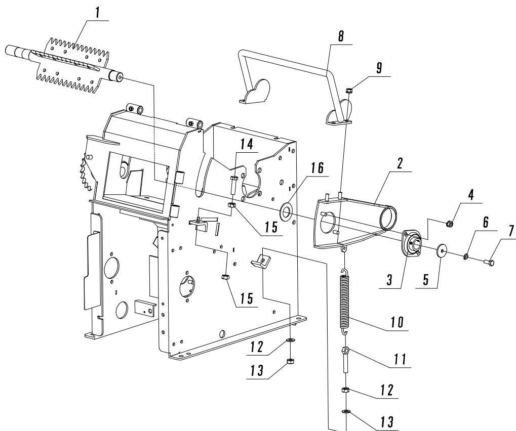
Fig. 20 フィードローラ①
