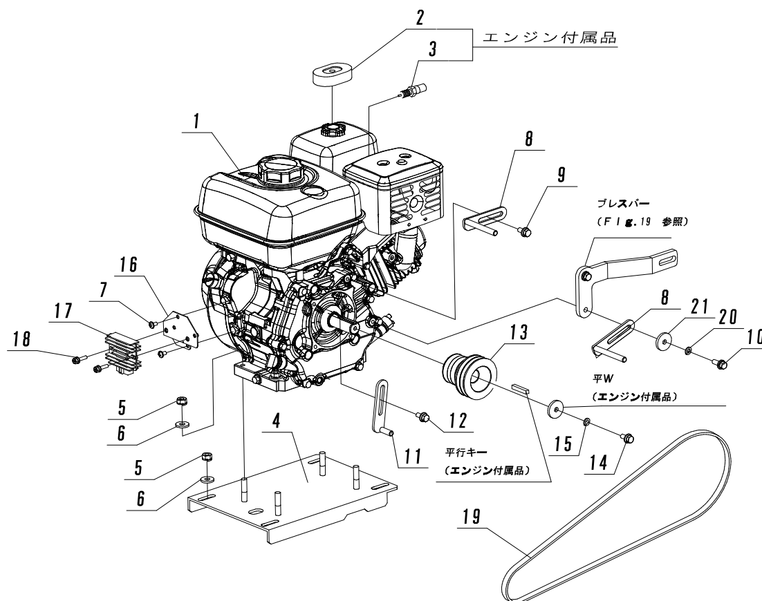
Fig. 9 エンジン
