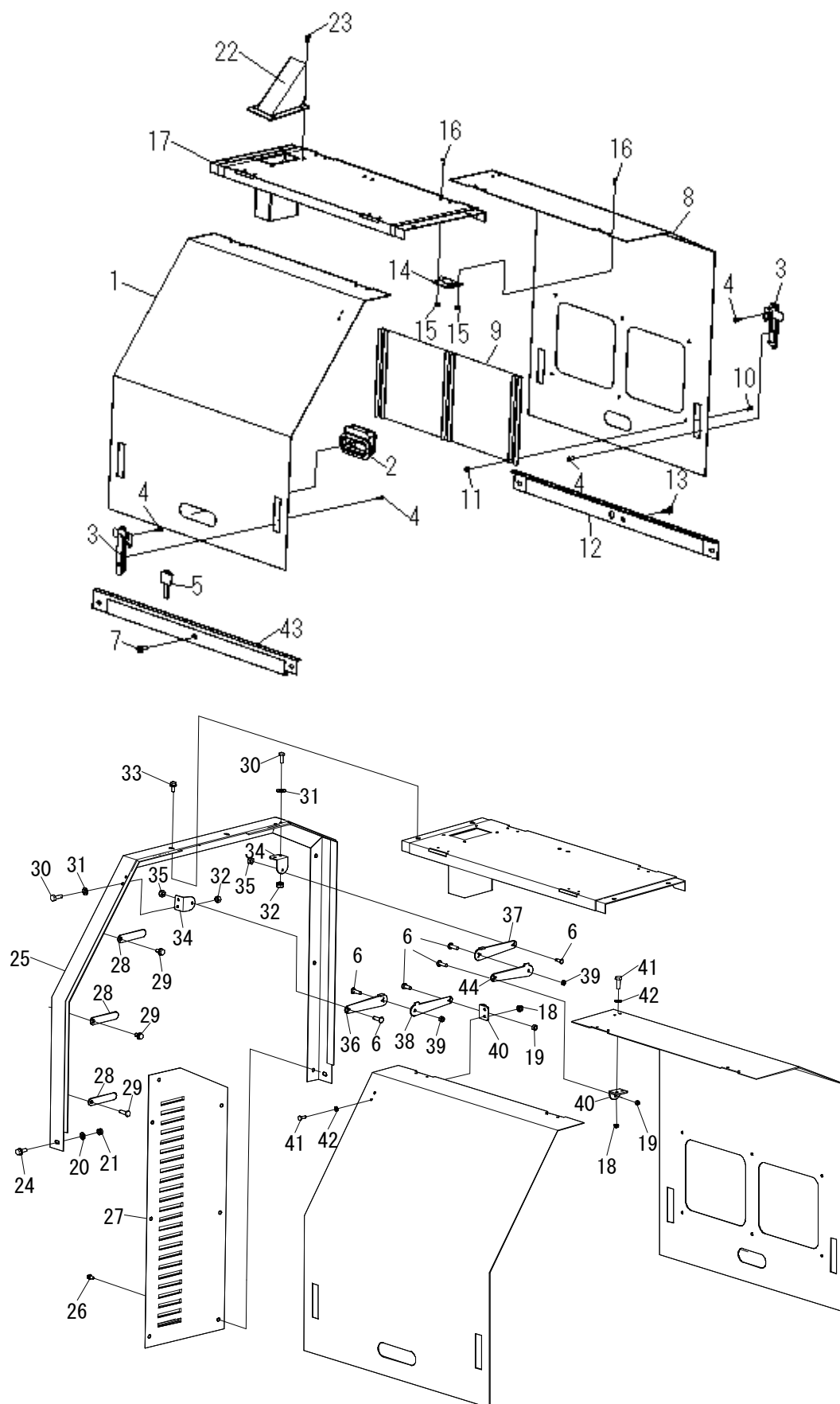
Fig. 17-2 カバー系
