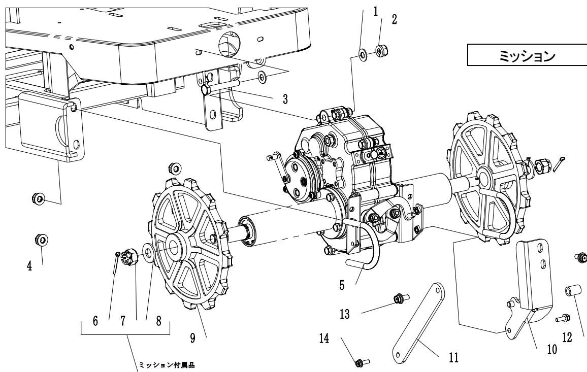
Fig. 3 フレーム(3)
