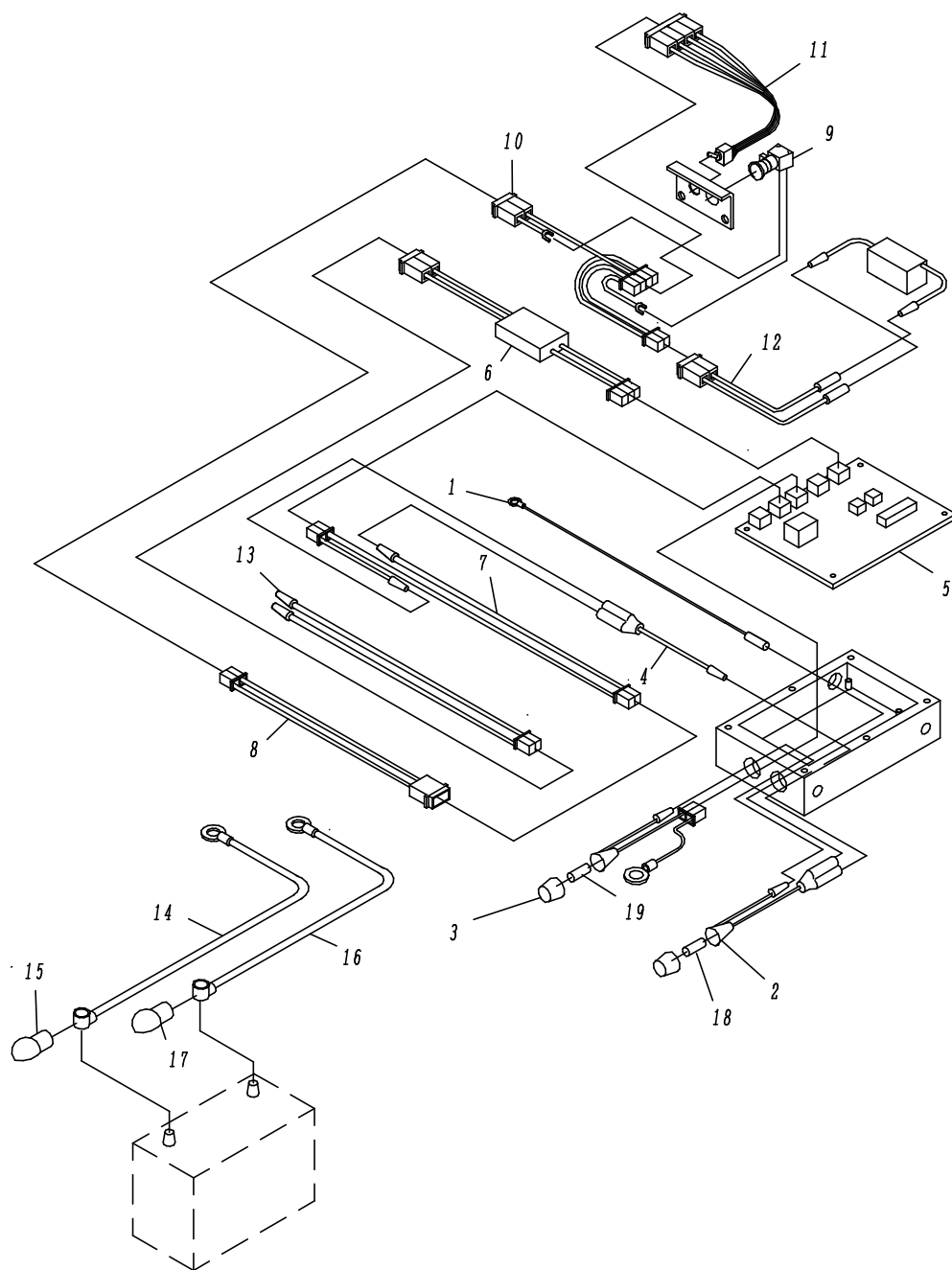
Fig. 9 配線系
