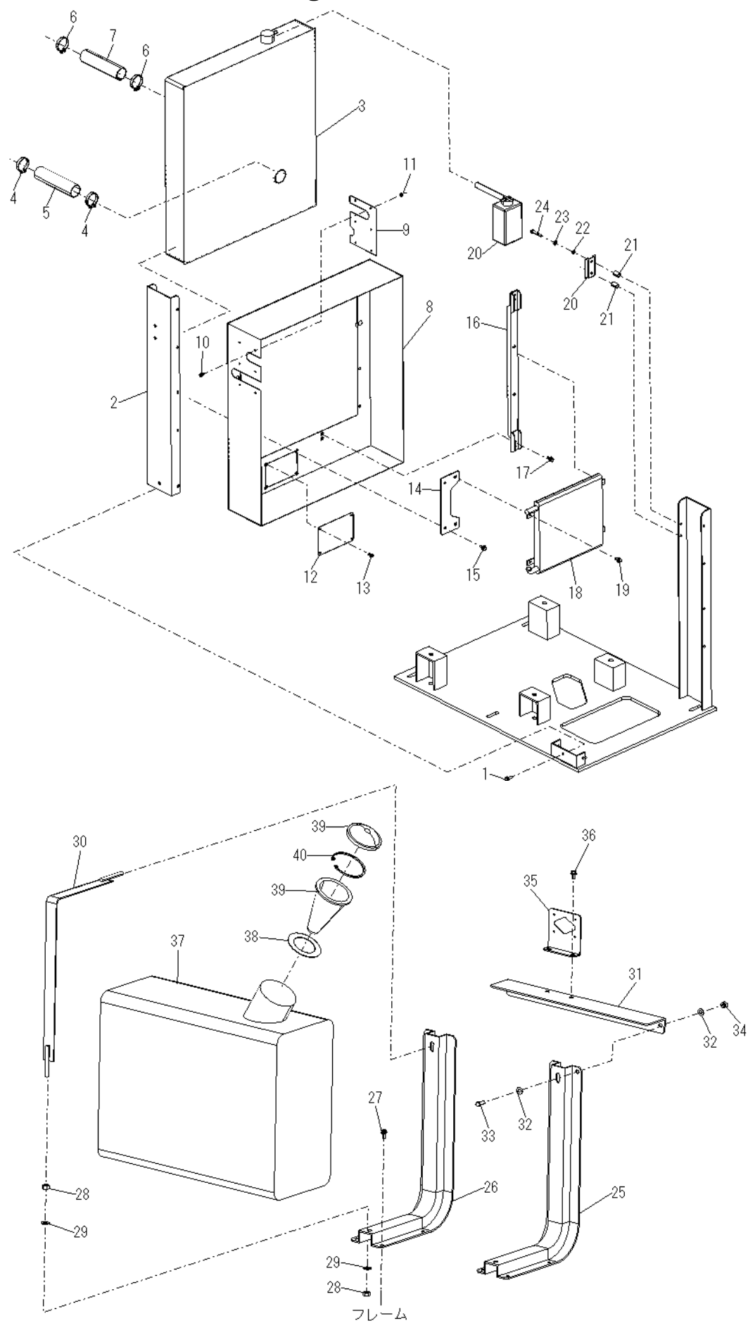
Fig. 3-1 エンジン系
