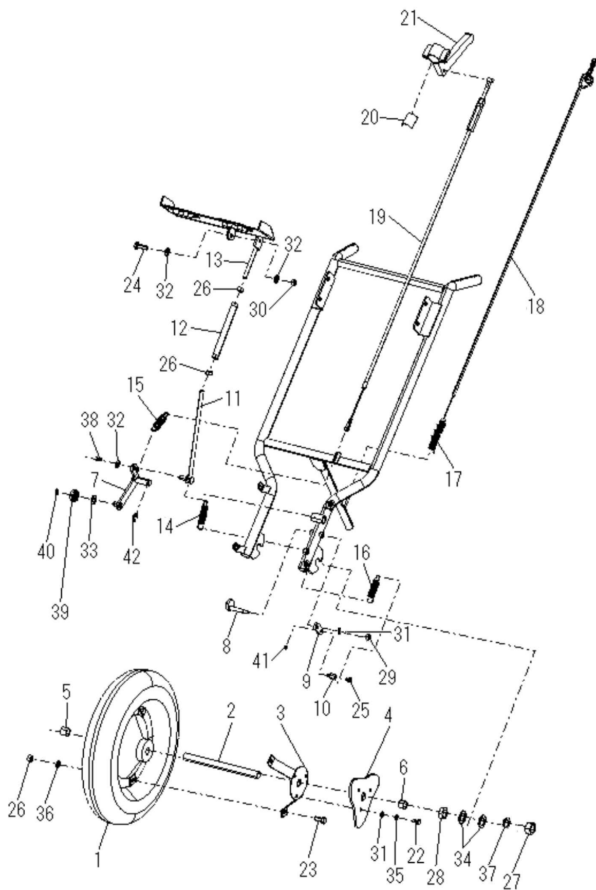
Fig. 4 1101600A000 駆動系
