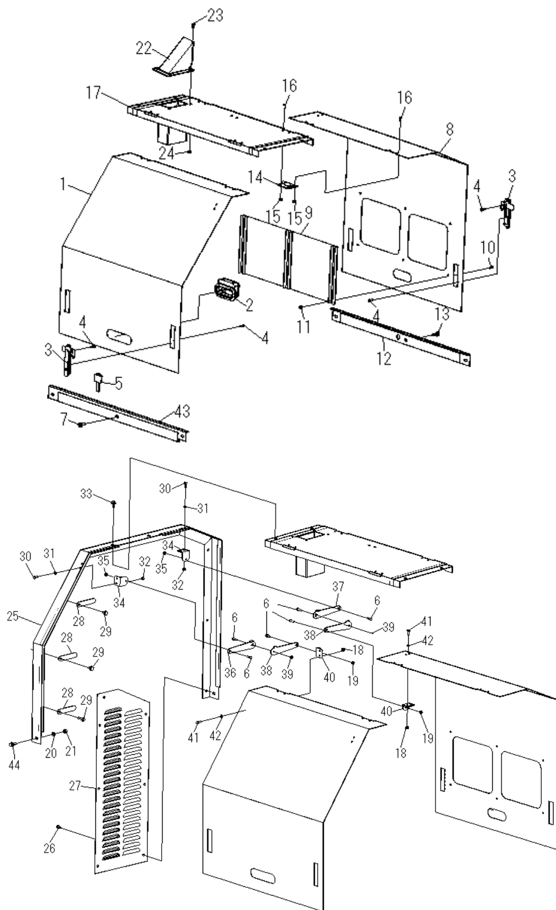
Fig. 17-2 カバー系
