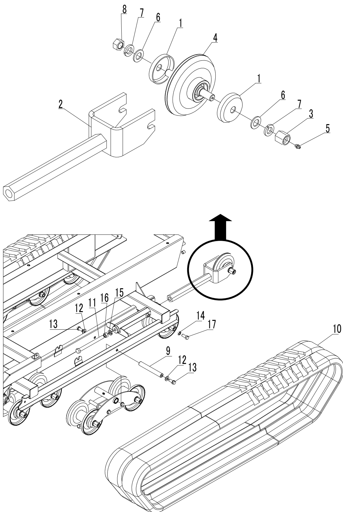
Fig. 3 誘導輪系
