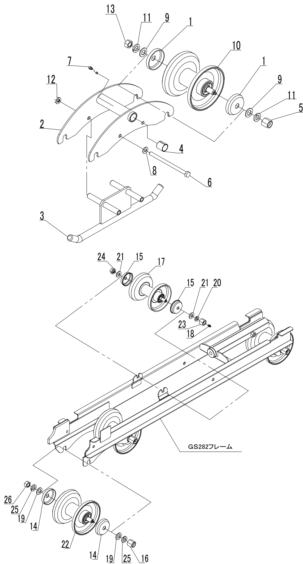
Fig. 2 転輪系
