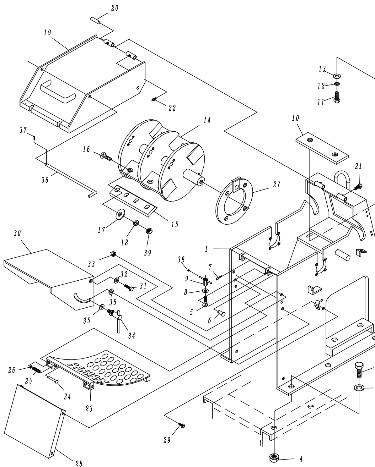
Fig. 6 ロータ系
