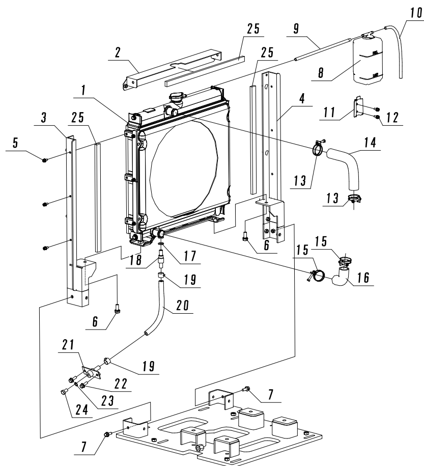
Fig. 18-5 エンジン⑤
