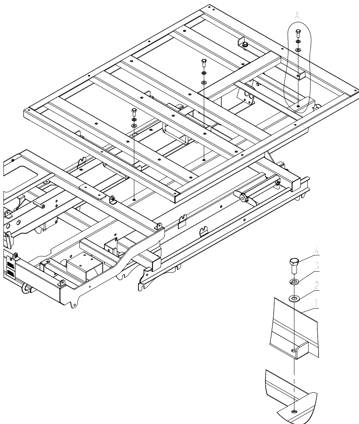
Fig. 11 ベースフレーム取付
