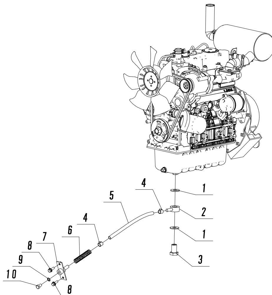
Fig. 18-7 エンジン⑦
