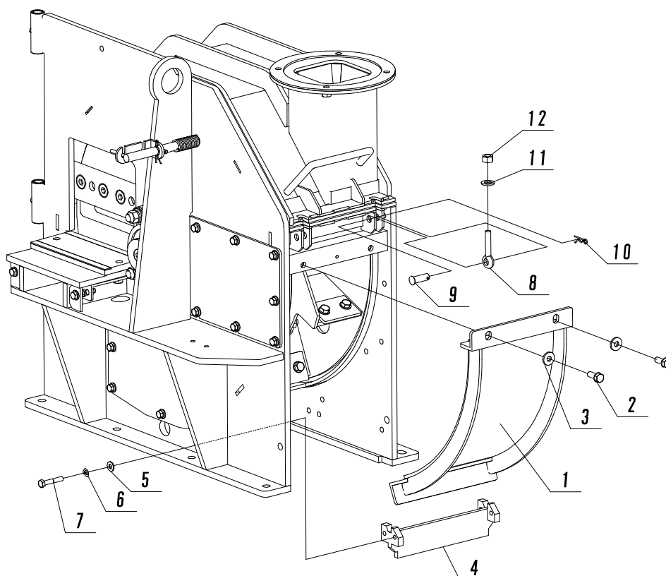
Fig. 27-2 ロータハウジング②
