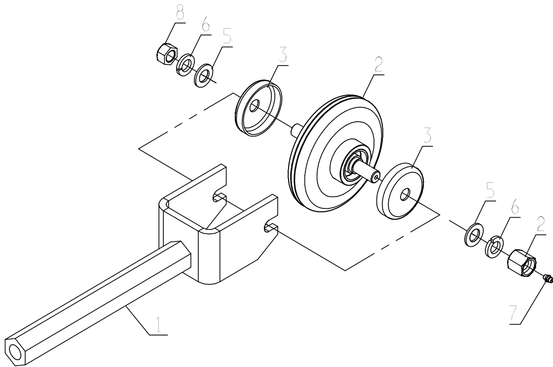
Fig. 3 誘導輪Sub組
