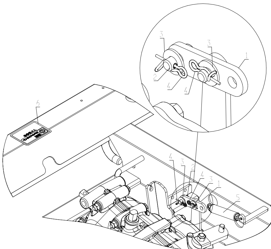
Fig. 9 連結ブラケット取付
