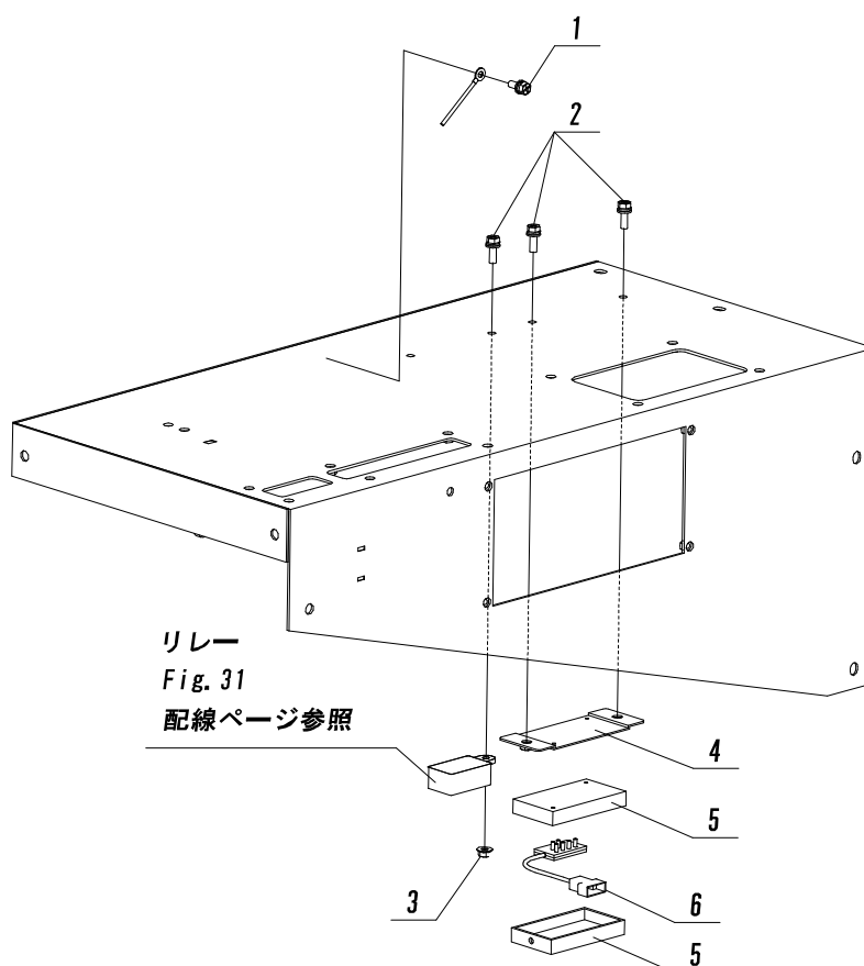
Fig. 21 シリンダコントロール
