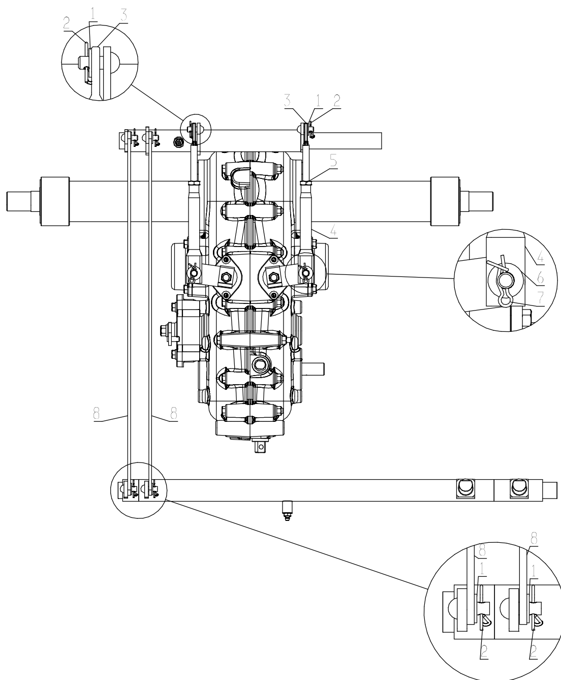
Fig. 8 サイドクラッチBK取付
