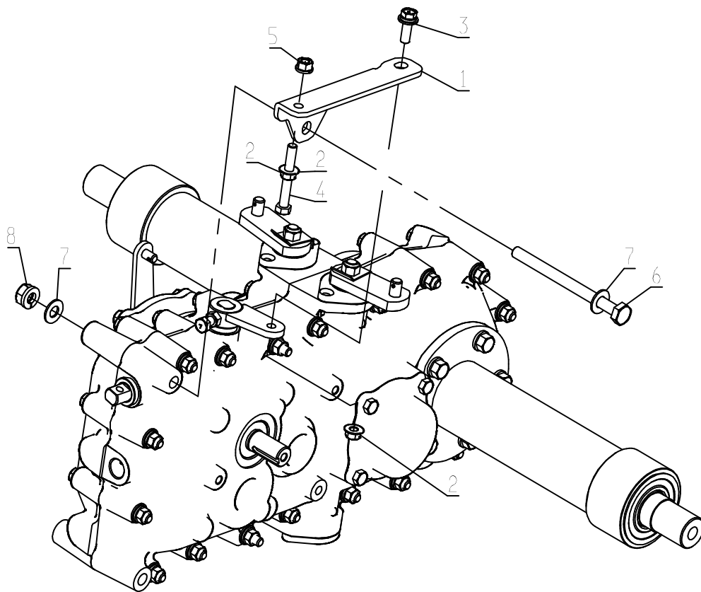
Fig. 1-2 ミッションSub組
