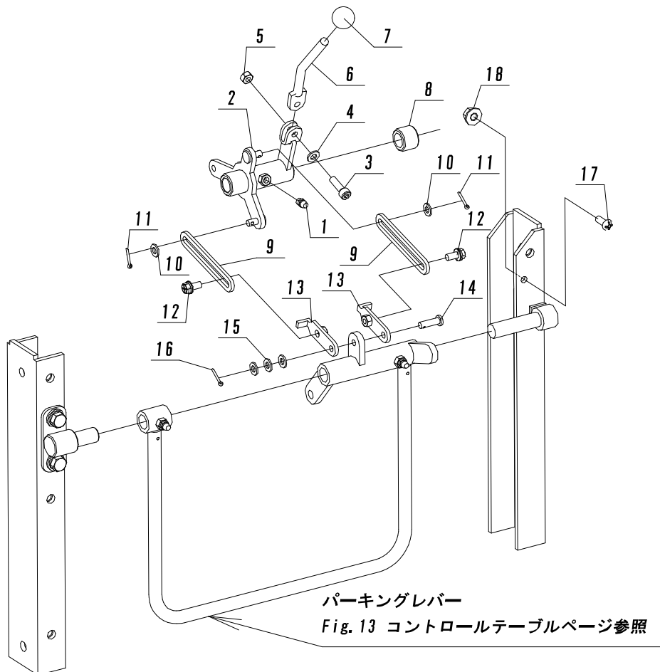
Fig. 14-1 オペレーションアーム①
