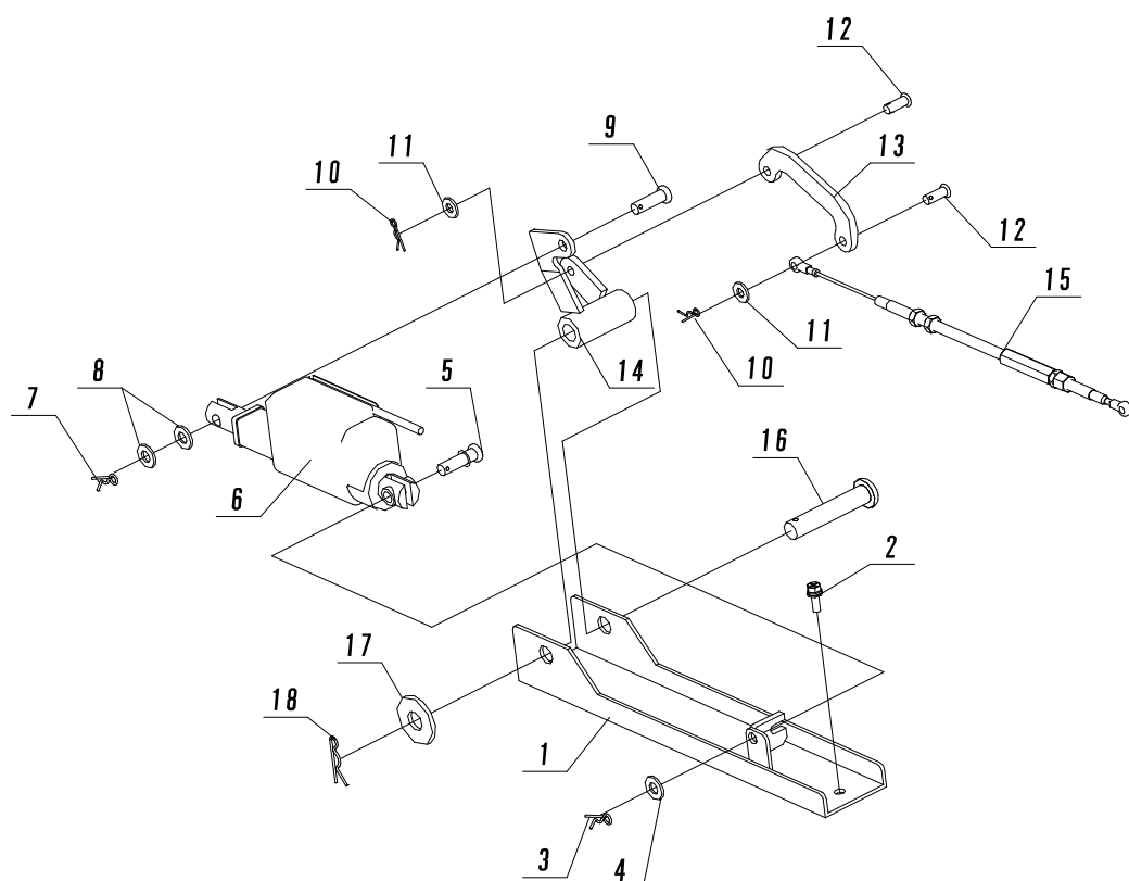
Fig. 20 アクチュエータ
