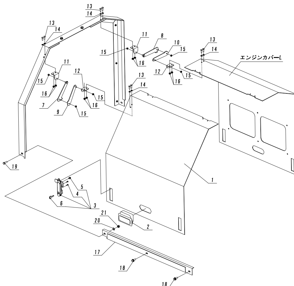
Fig. 30-3 カバー③
