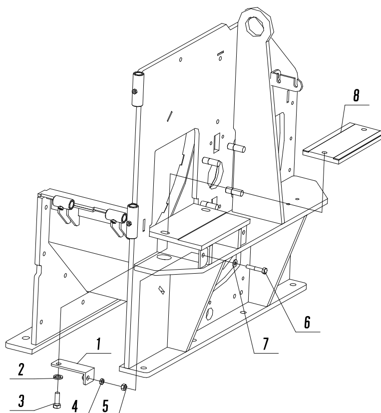
Fig. 26 受刃
