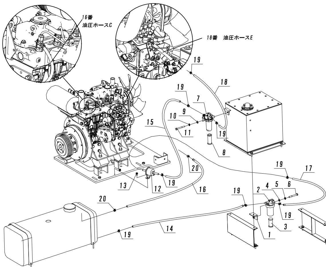
Fig. 19-2 燃料タンク②
