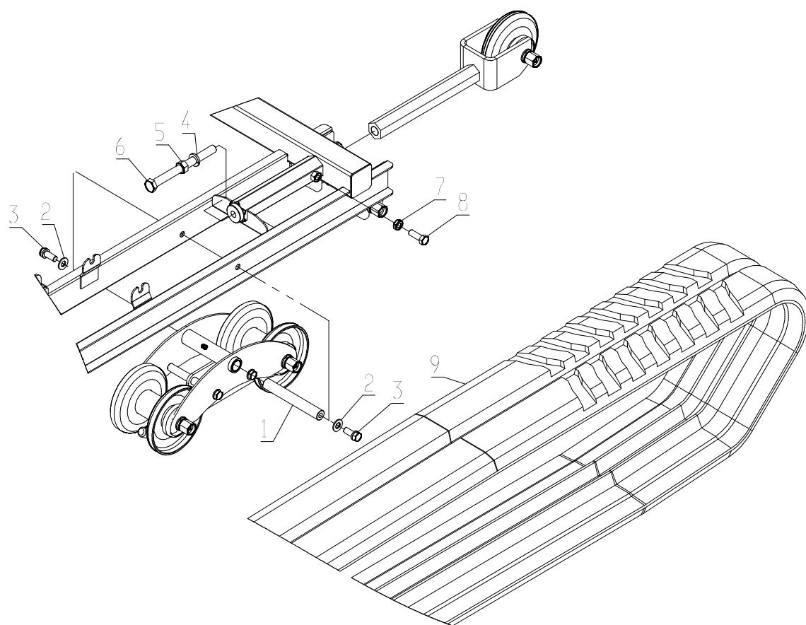
Fig. 6 クローラ取付
