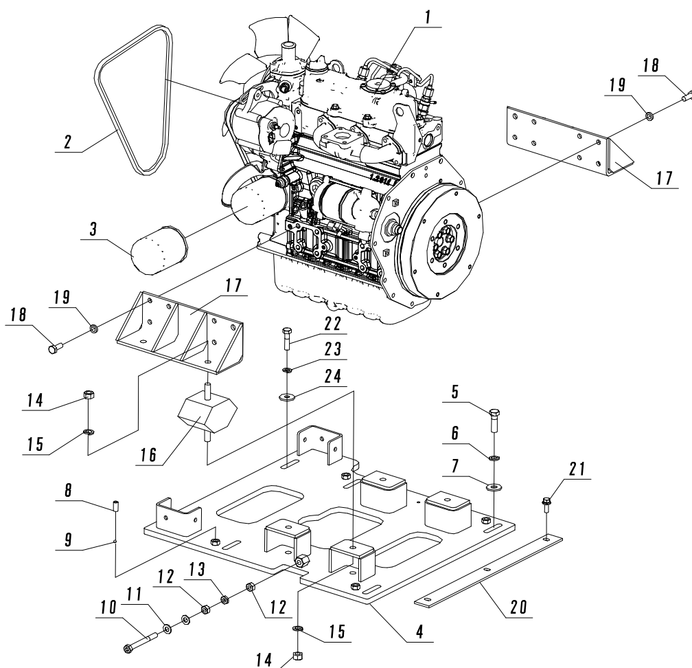
Fig. 18-1 エンジン①
