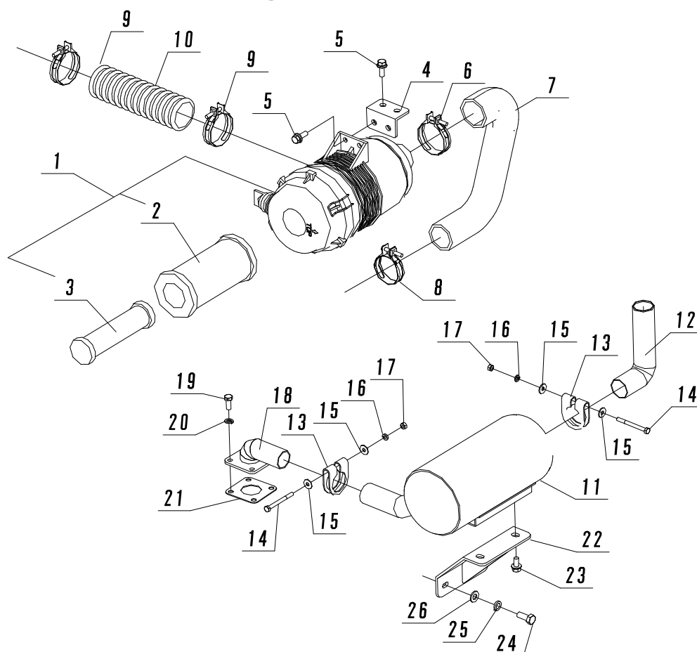
Fig. 18-4 エンジン④
