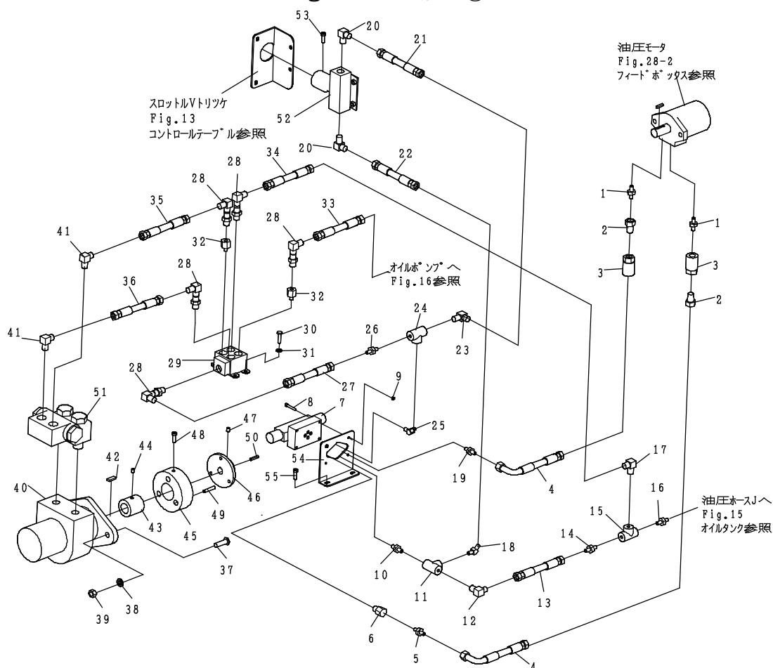
Fig. 17-2 油圧②
