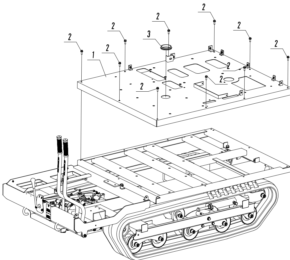
Fig. 12 ベースフレーム
