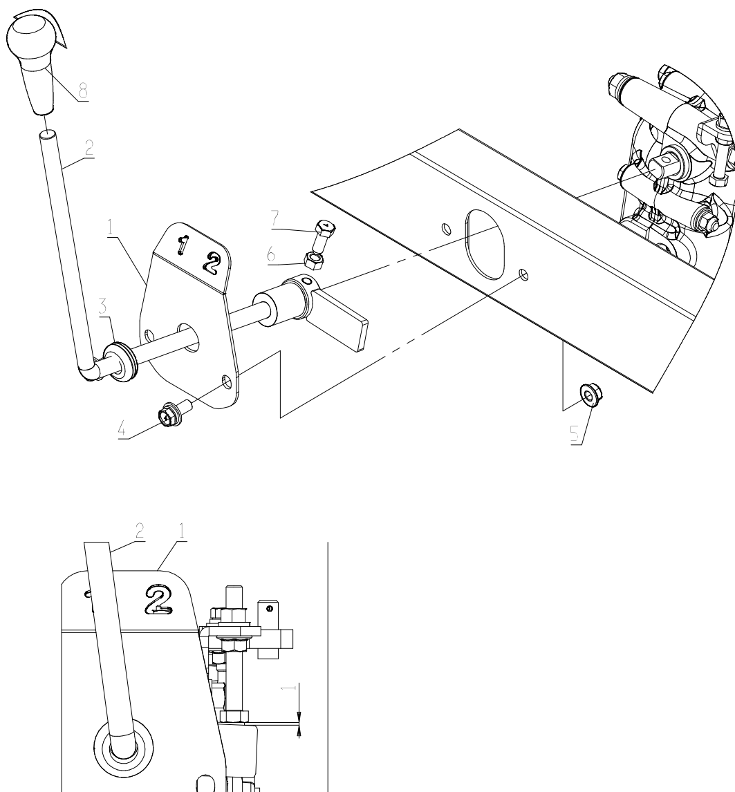
Fig. 10 チェンジレバー取付
