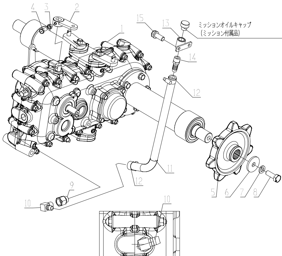
Fig. 1-1 ミッションSub組
