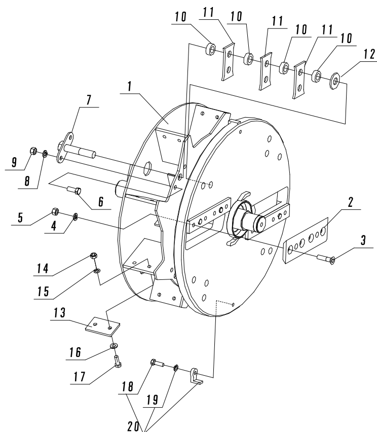
Fig. 25 ロータジク、チツパナイフ
