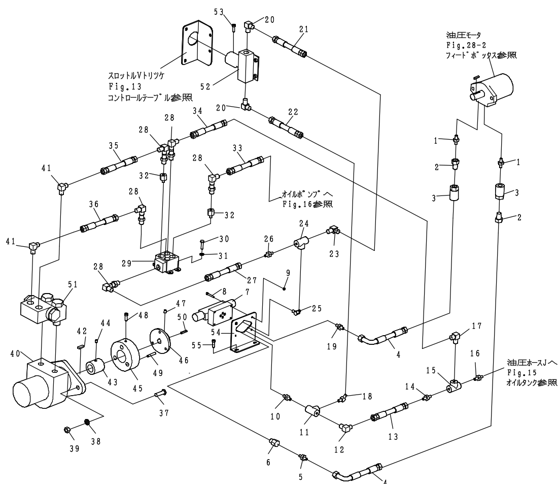
Fig. 17-1 油圧①
