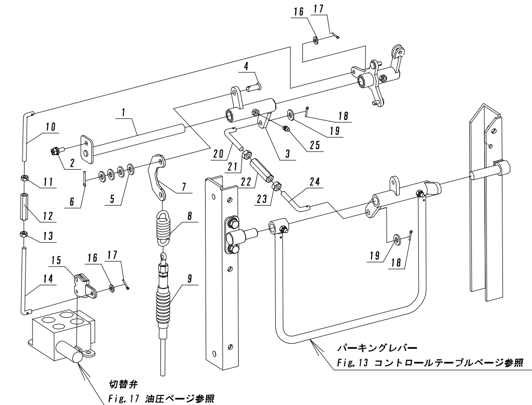
Fig. 14-2 オペレーションアーム②
