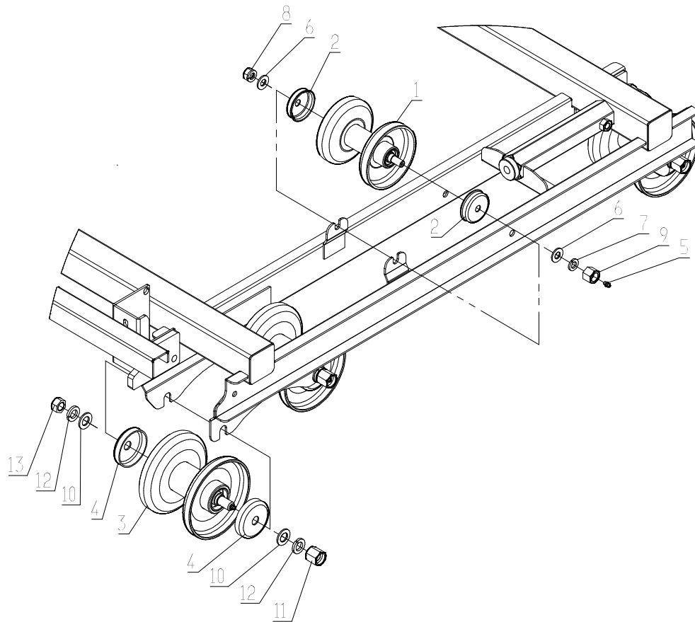
Fig. 5 転輪取付
