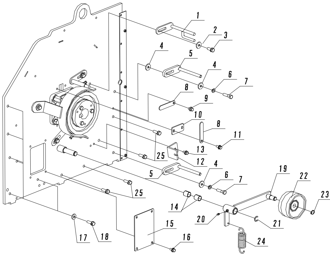
Fig. 24-2 RHサイドプレートF②
