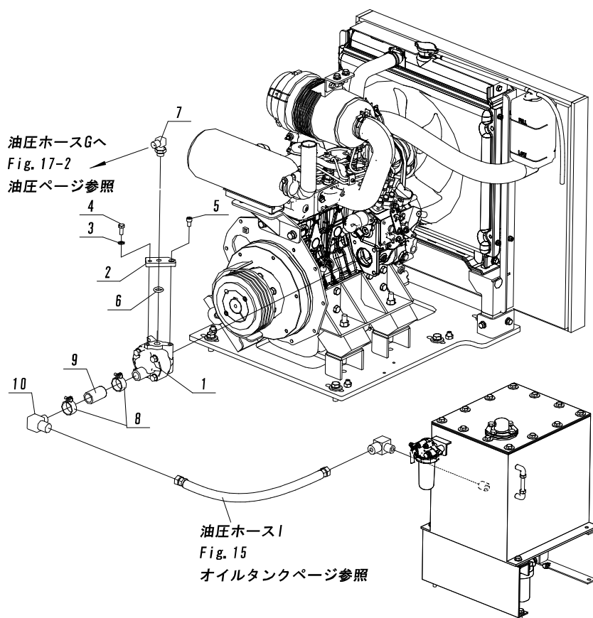
Fig. 16 オイルポンプ
