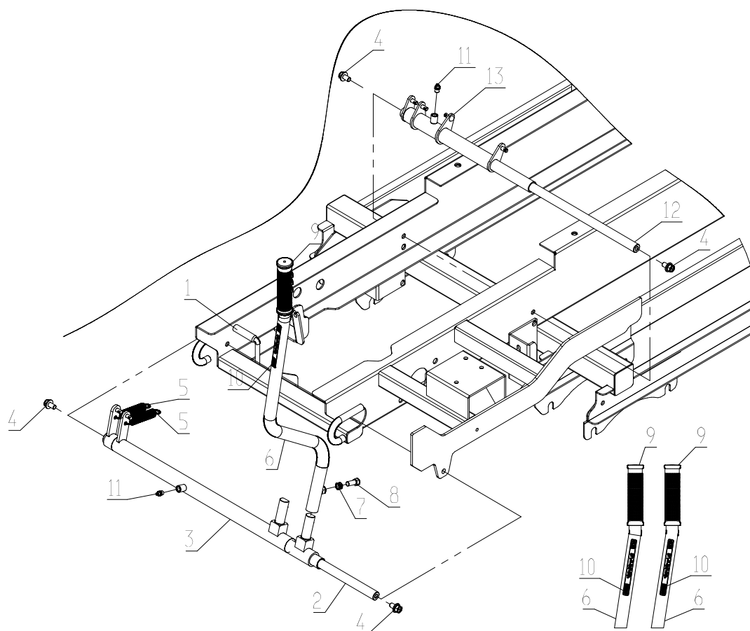
Fig. 7 サイドクラッチリンク取付
