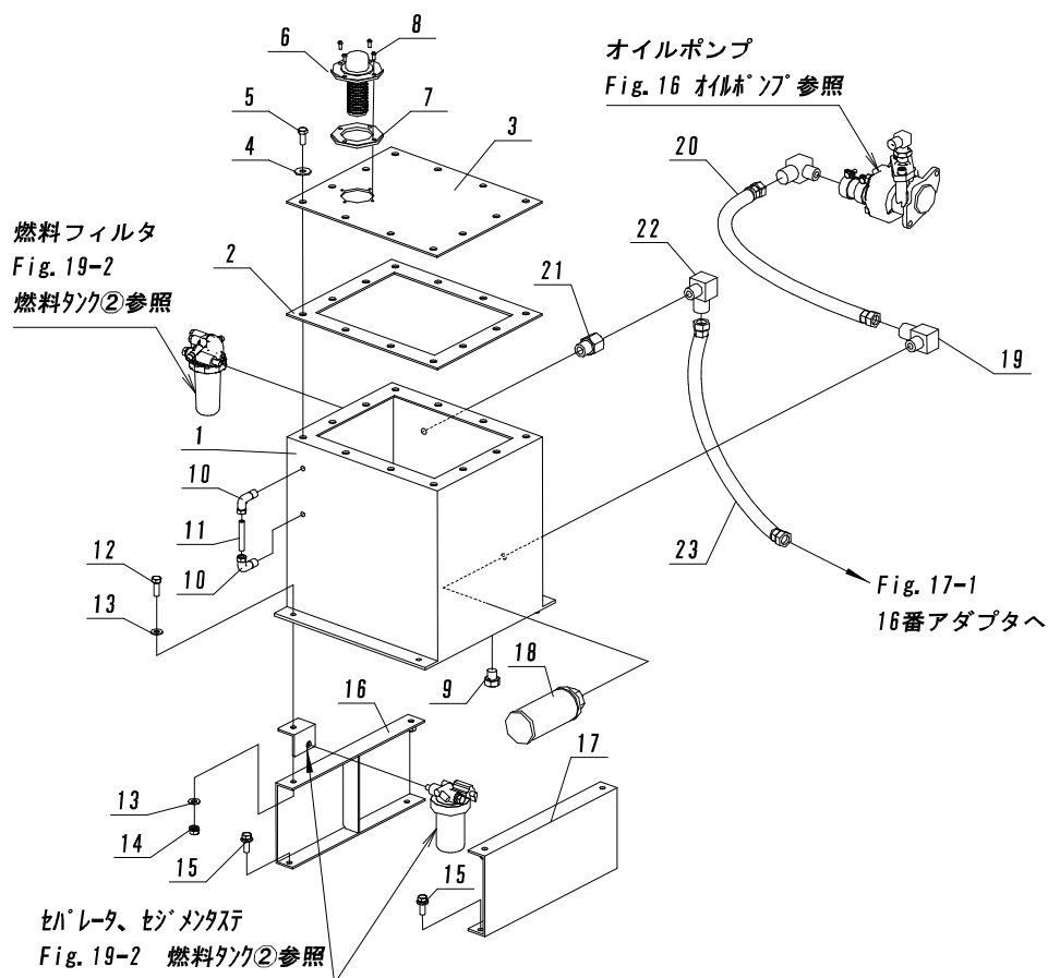
Fig. 15 オイルタンク
