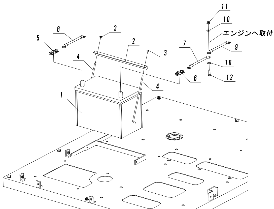
Fig. 23 バッテリ
