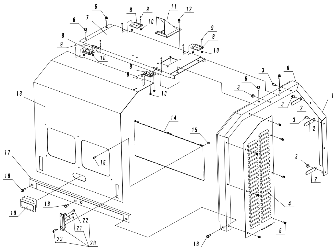
Fig. 30-2 カバー②
