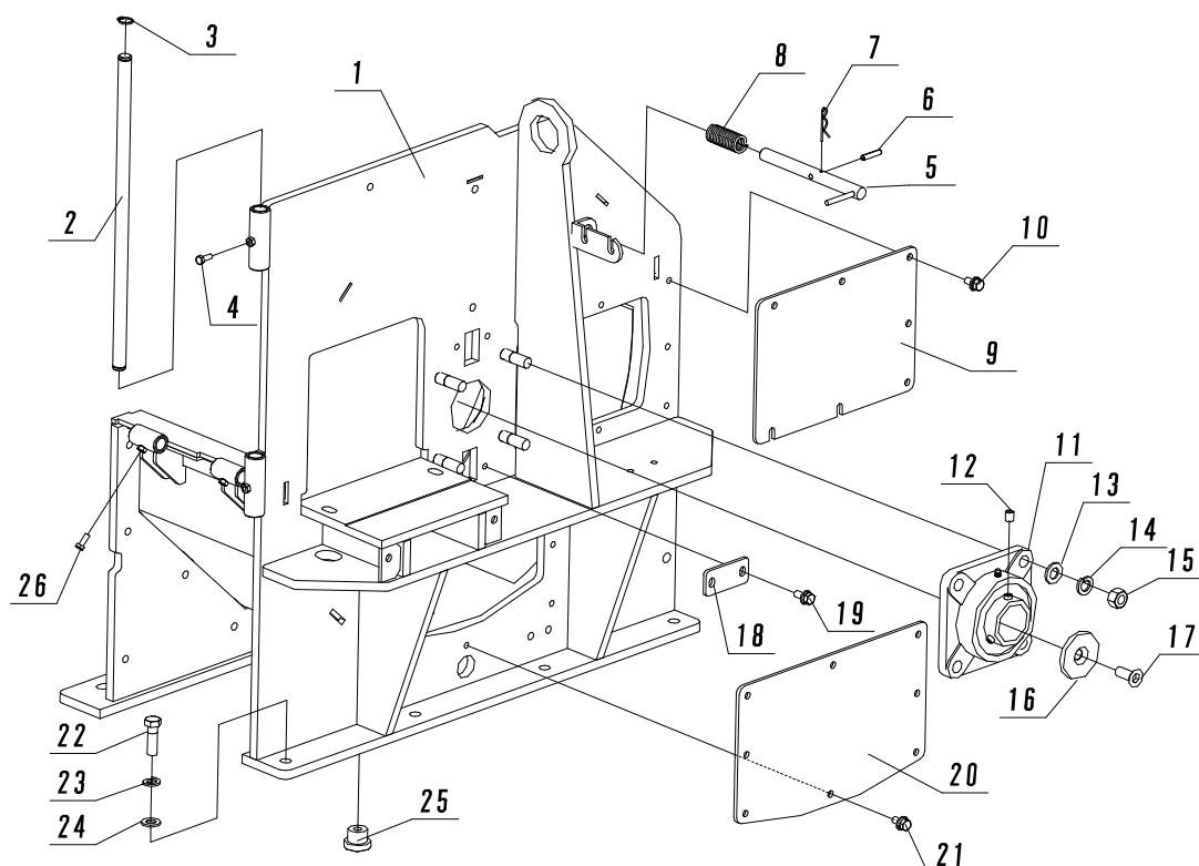
Fig. 27-1 ロータハウジング①
