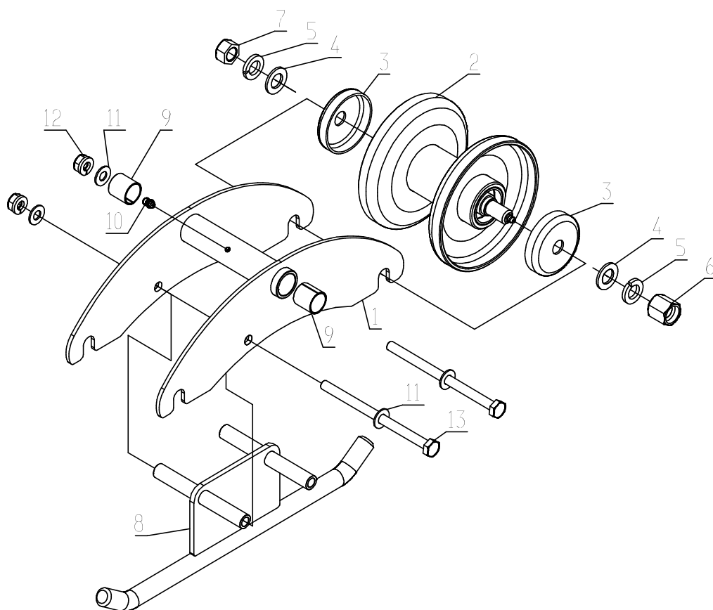
Fig. 2 イコライザーSub組
