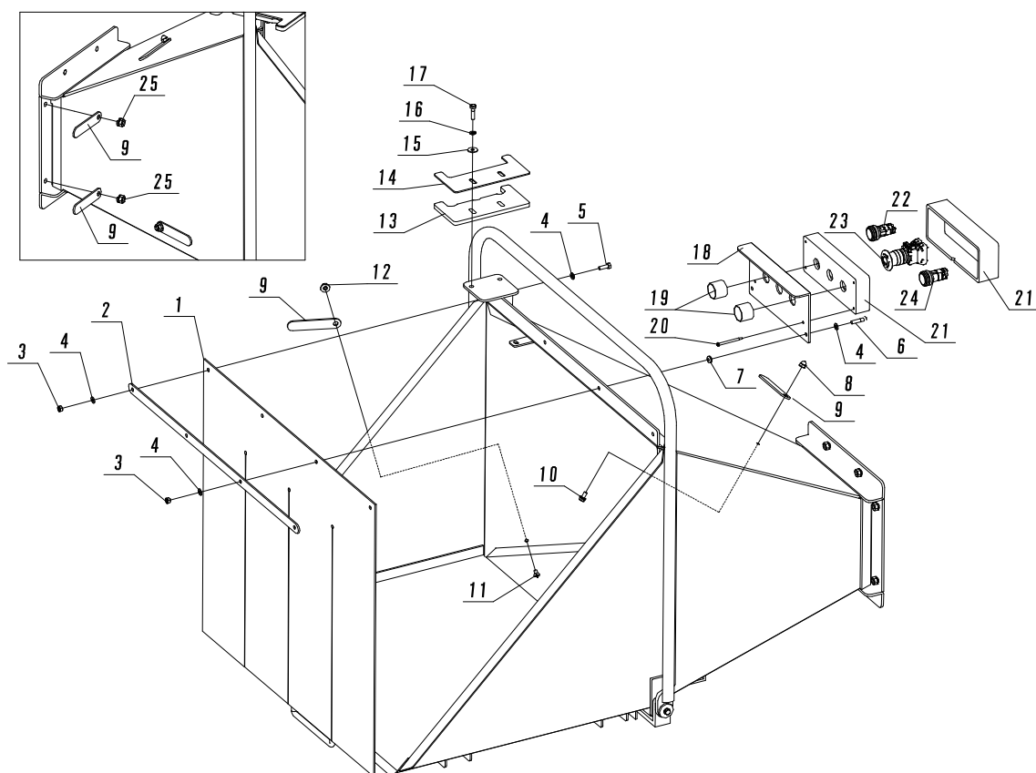
Fig. 29-2 ホツパ②
