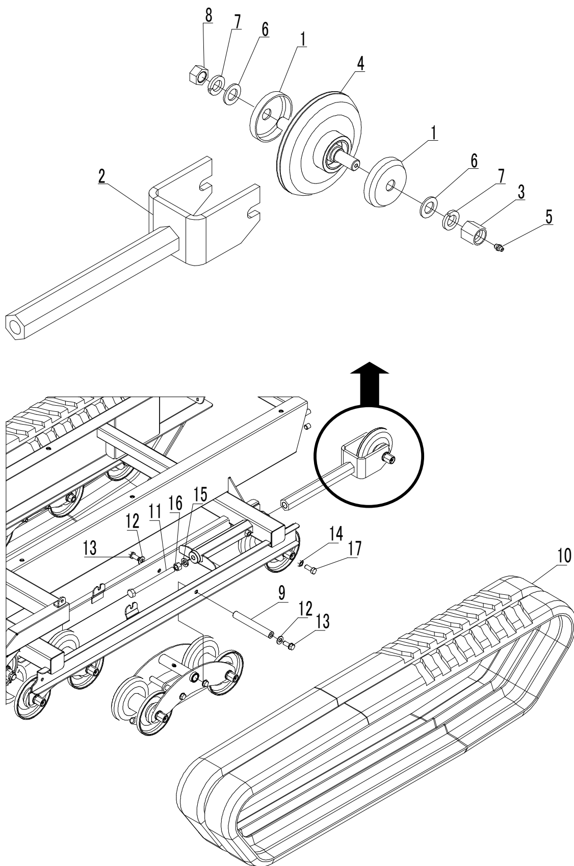
Fig. 3 誘導輪系
