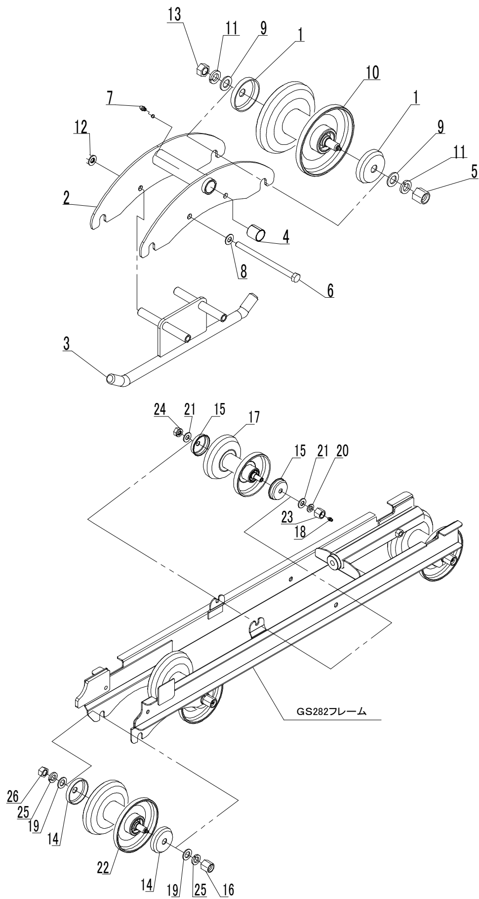
Fig. 2 転輪系
