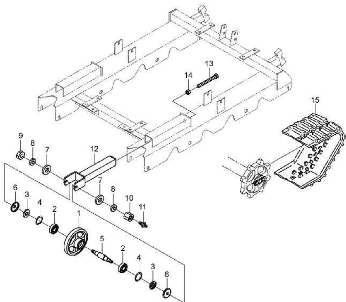
Fig. 9 クローラ系
