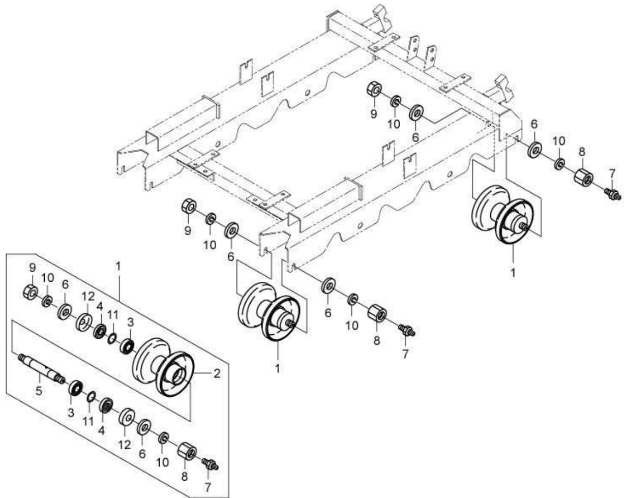
Fig. 6 転輪系(1)
