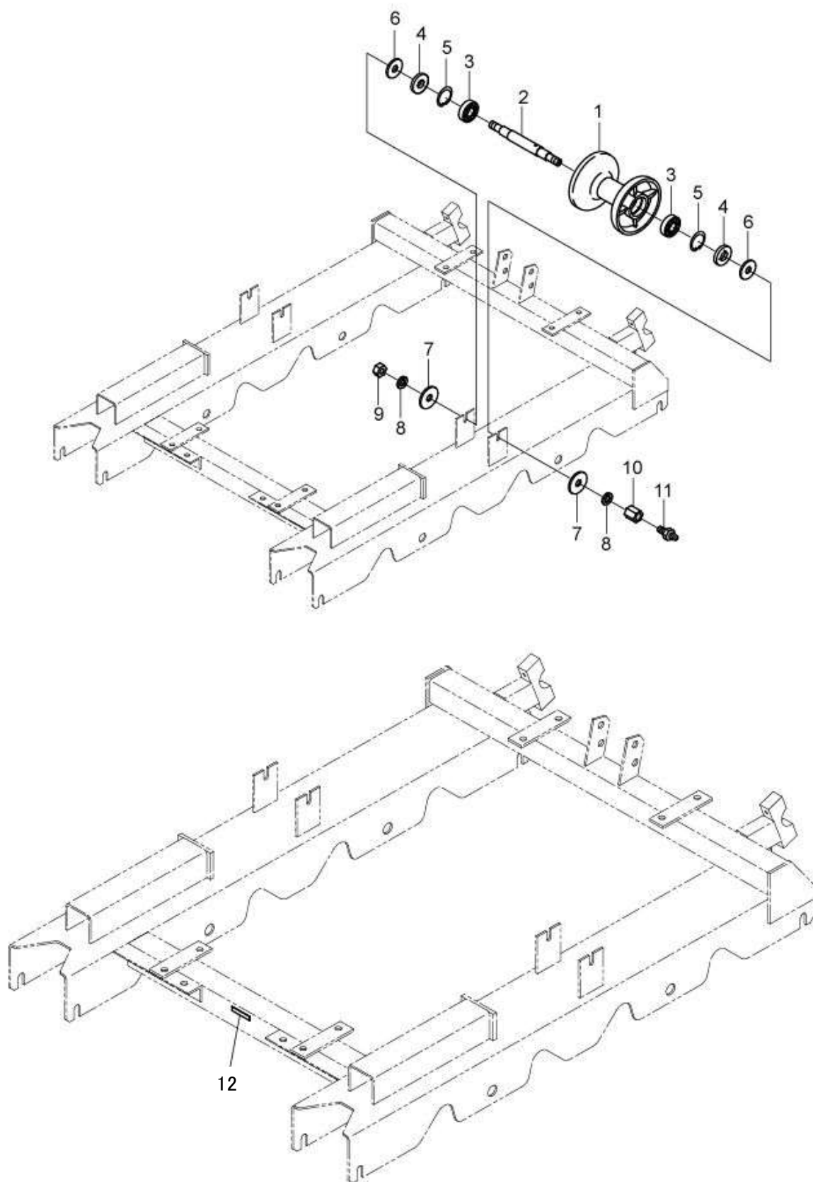
Fig. 8 転輪系(3)
