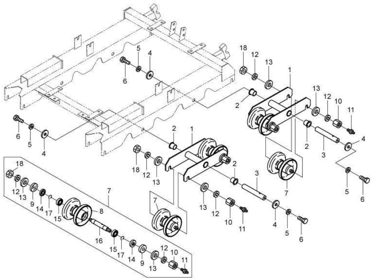
Fig. 7 転輪系(2)
