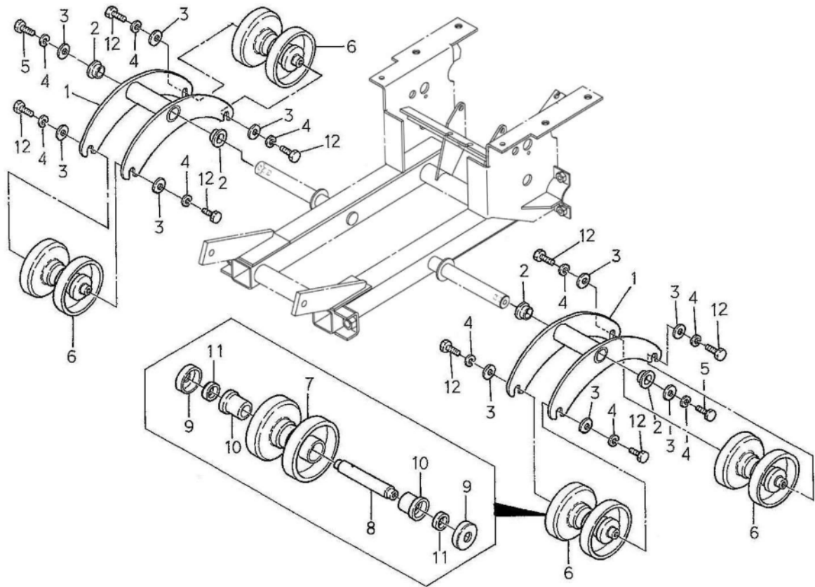
Fig.2 フレーム系(2)
