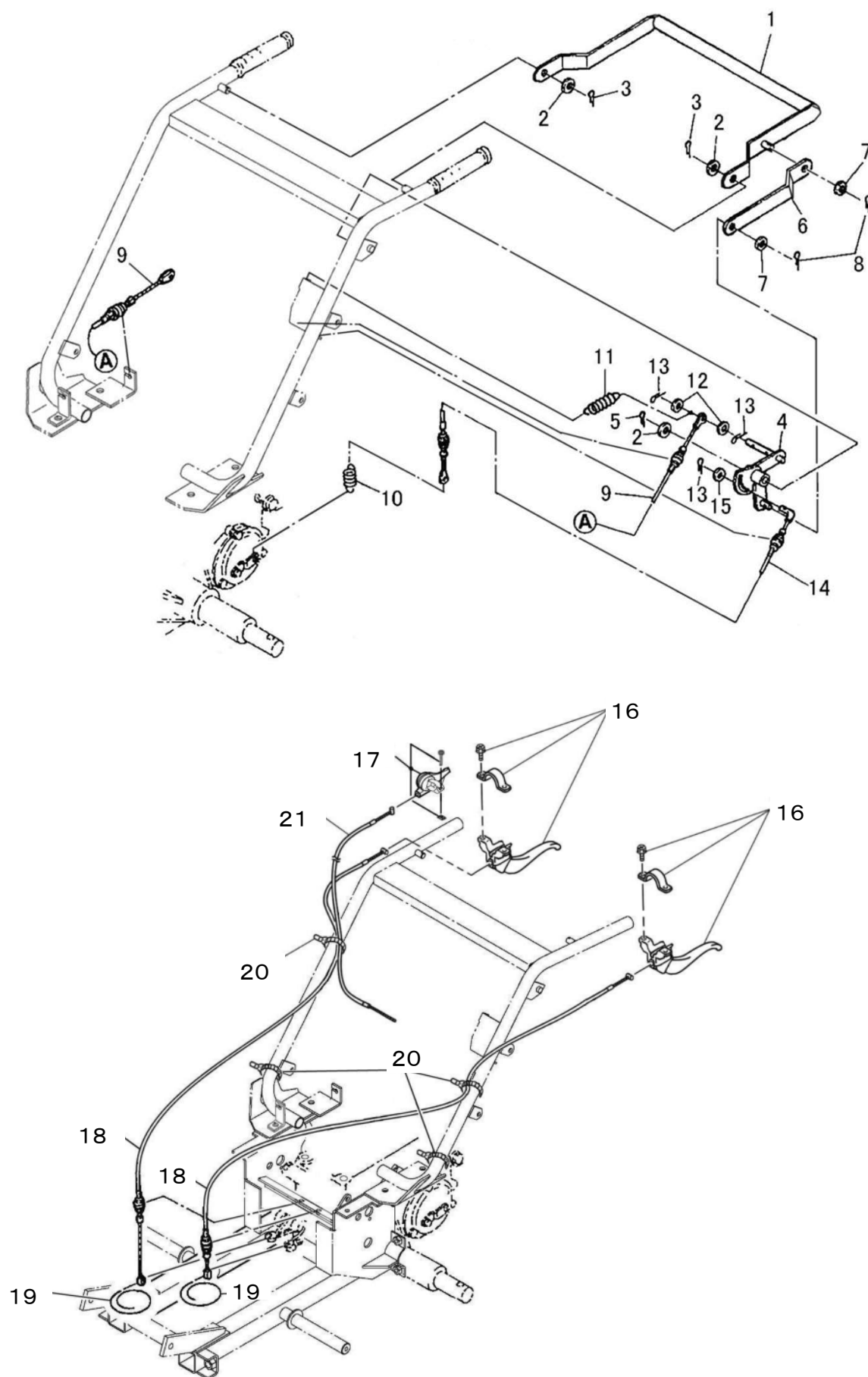
Fig.4 走行レバー系
