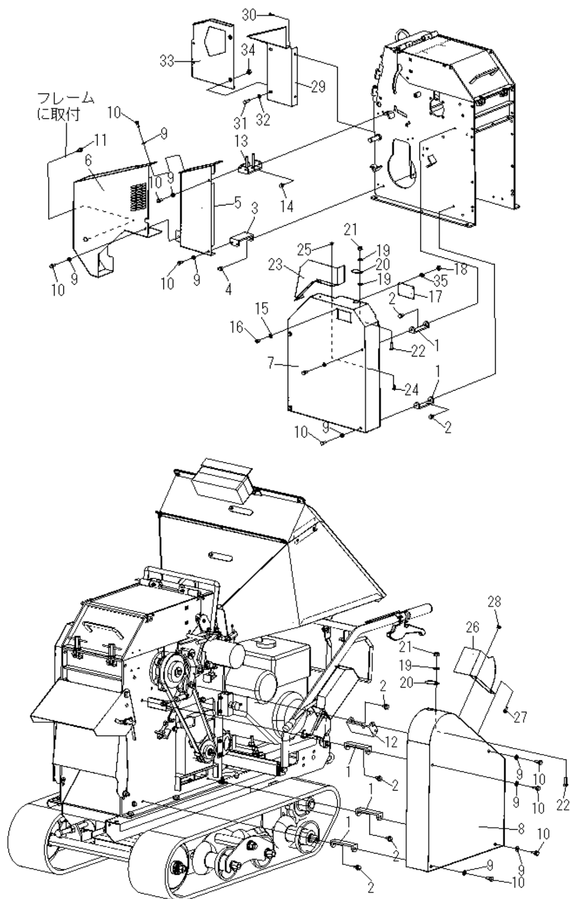
Fig. 10 カバー系
