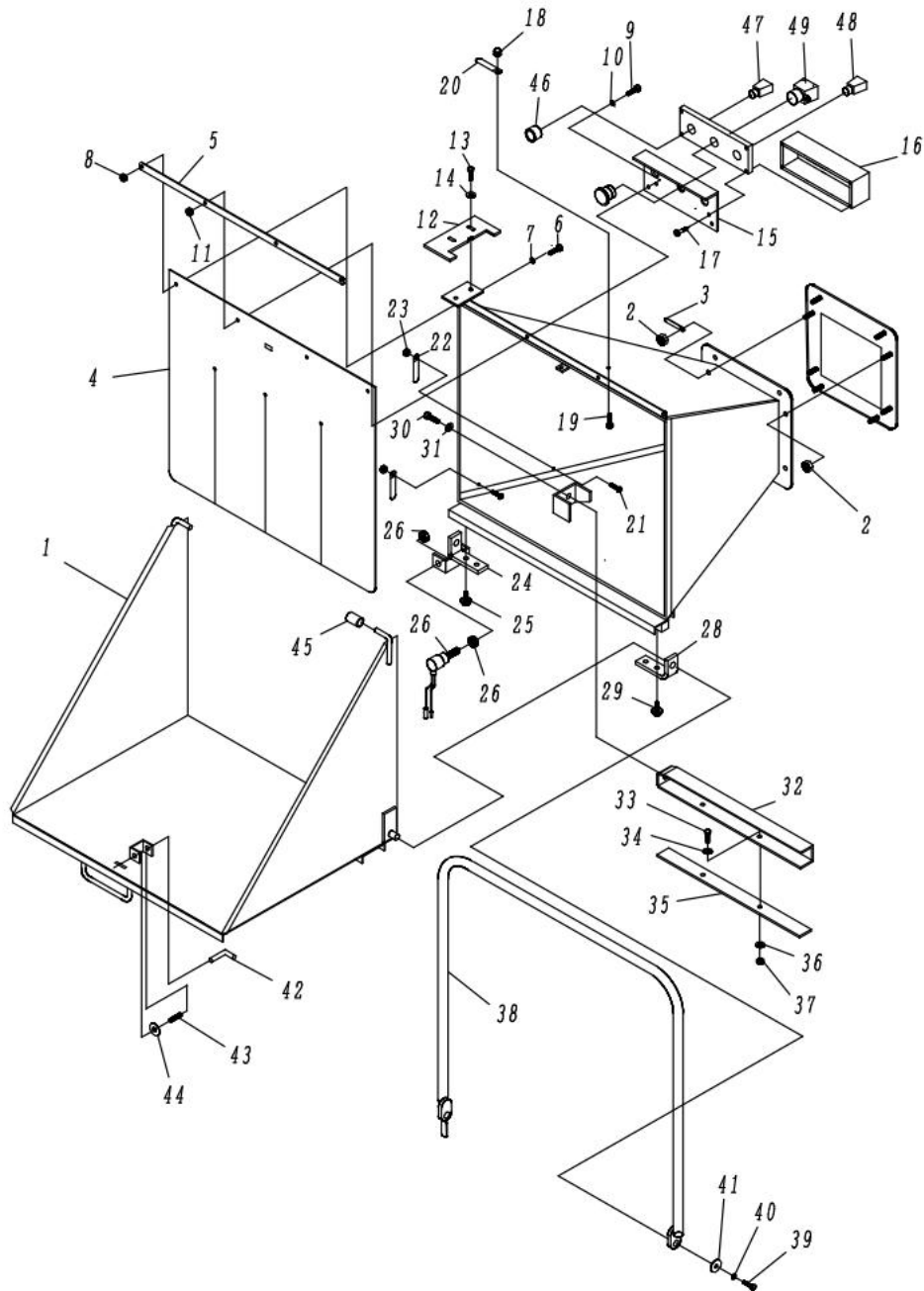
Fig. 8 ホツパ系
