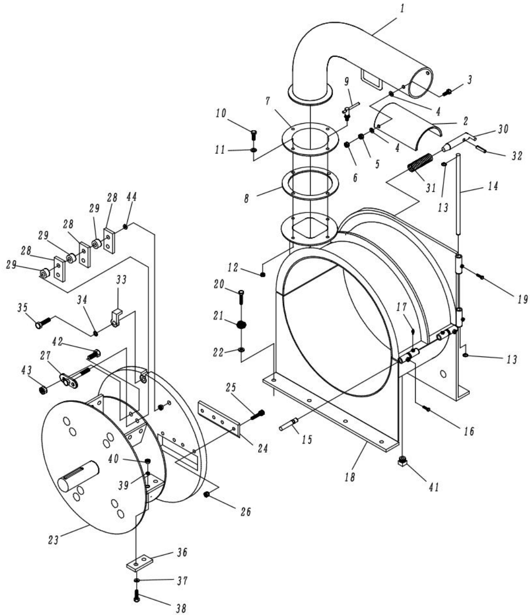
Fig. 6 ロータ系
