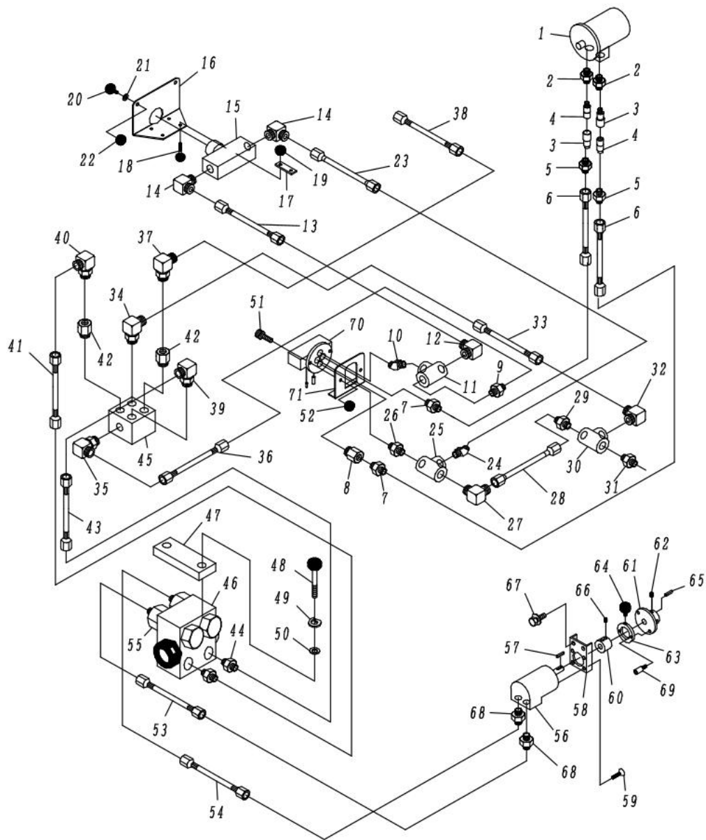
Fig. 3-1 油压系 (1)
