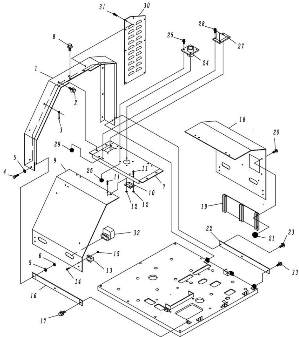
Fig. 9-1 カバー系
