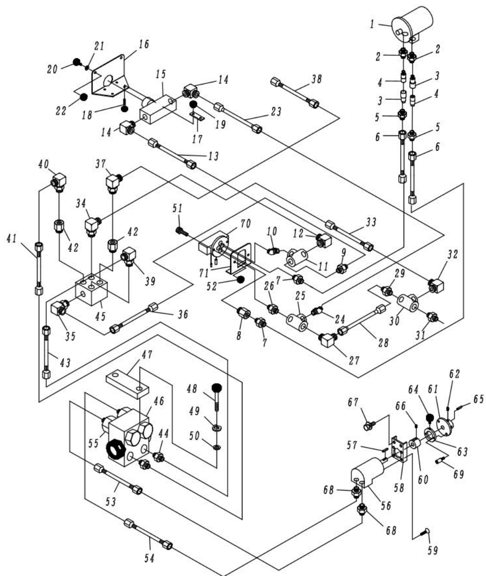
Fig. 3-1 油压系 (2)
