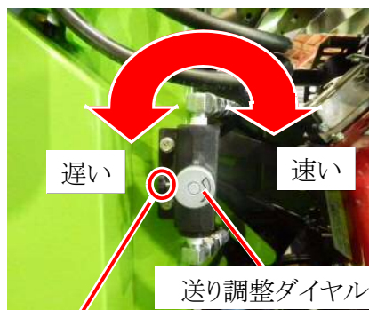
ダイヤルロックピン
