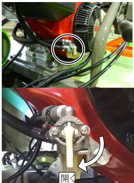
燃料コック
