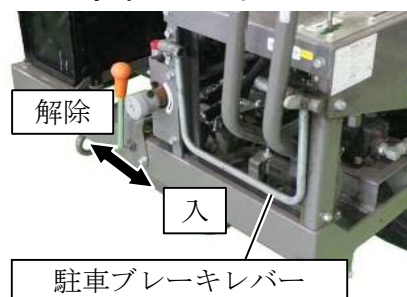
駐車ブレーキレバー
