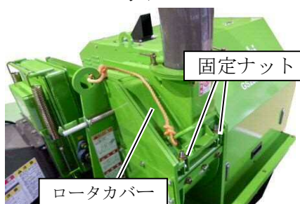
ロータカバー
