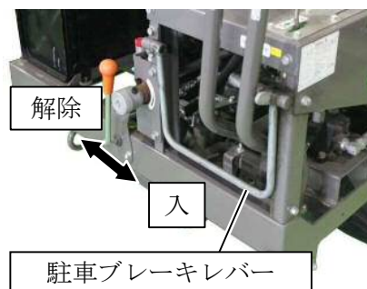
駐車ブレーキレバー
