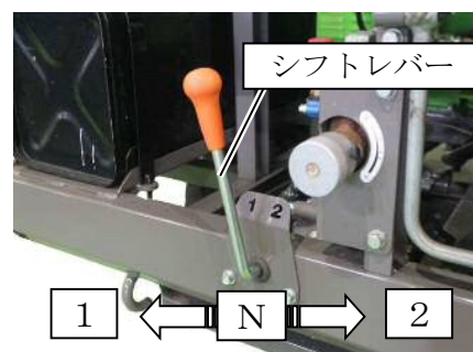
シフトレバー
