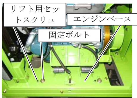
エンジンベース
