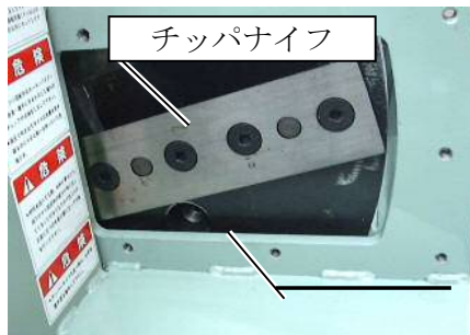
点検窓
