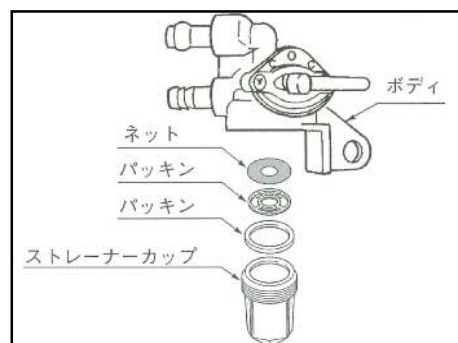
燃料コック
