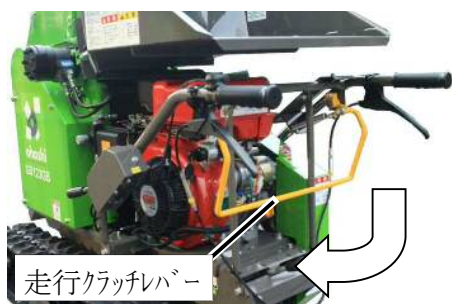
走行クラッチレバー
