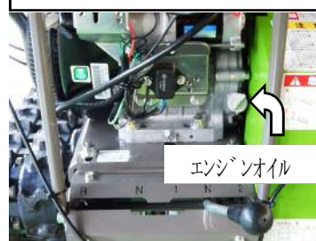
エンジン
