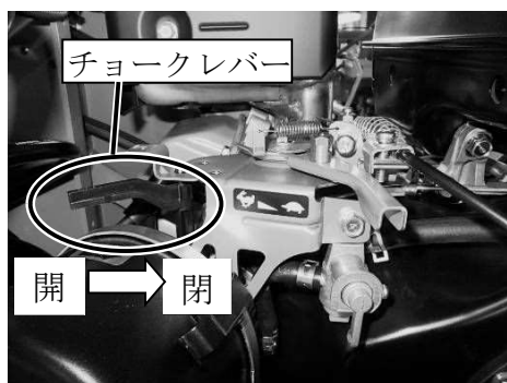
エンジン
